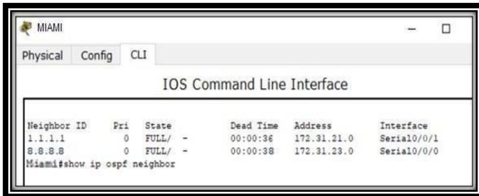
Figura 20 Verificación Miami conectado por OSPFv2
