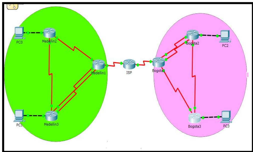
Figura 2 Topología Escenario 1 en packet tracer
