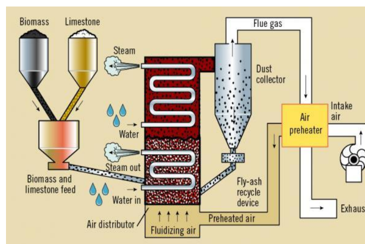
Figura 5. Caldera de lecho fluidizado Fuente: Becerra. (2017)
