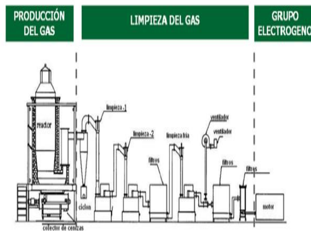
Figura 4. Esquema general de la gasificación. Fuente: Lesme, García, Ruiz, Pajarín, Revilla (2014)
