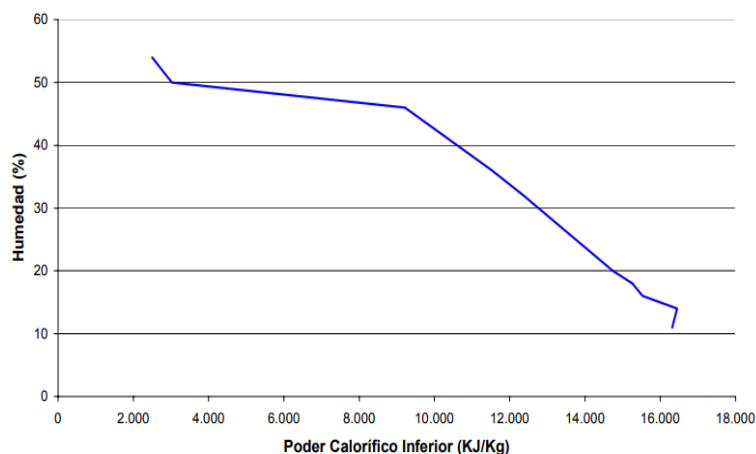
Figura 7. Variación del poder calorífico de la madera en función de la humedad. Fuente: Acer agroforestal (s.f)
