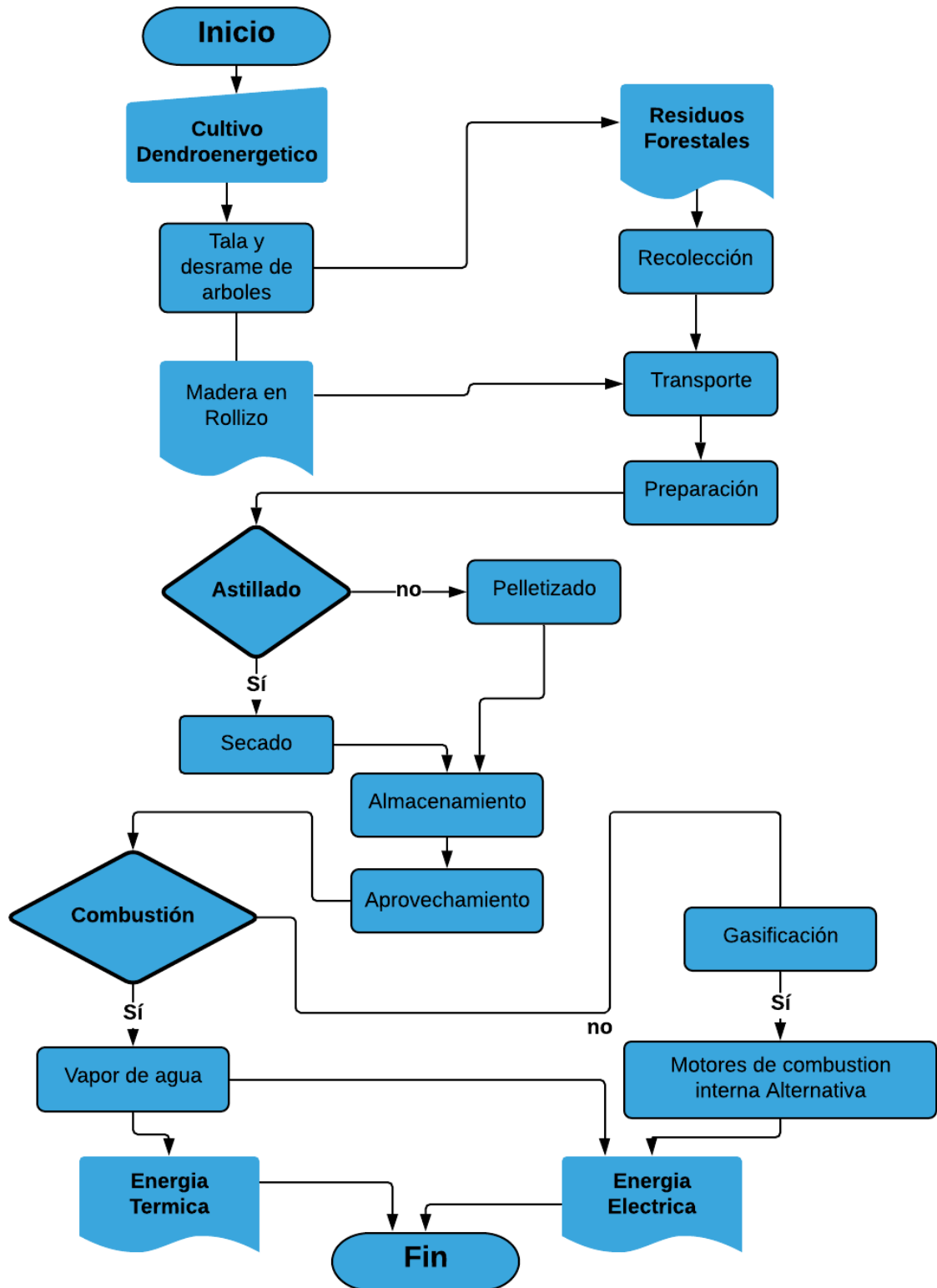
Figura 11. Diagrama de flujo ciclo de aprovechamiento de la biomasa
