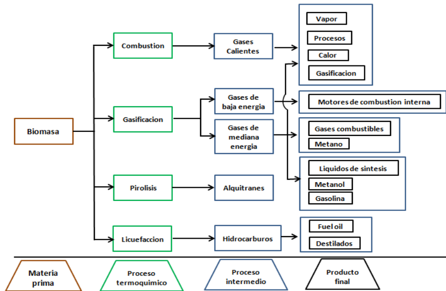
Figura 6. Esquema general de la gasificación. Fuente: Lesme, García, Ruiz, Pajarin, Revilla (2014)
