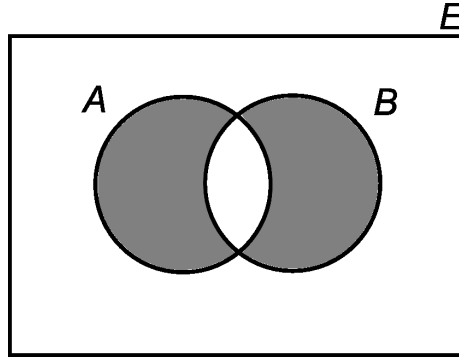
Figura 2.6: Representación gráfica del conjunto A \triangle B .
