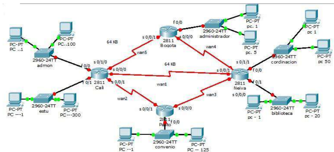
Figura 11. Topología UNAD
