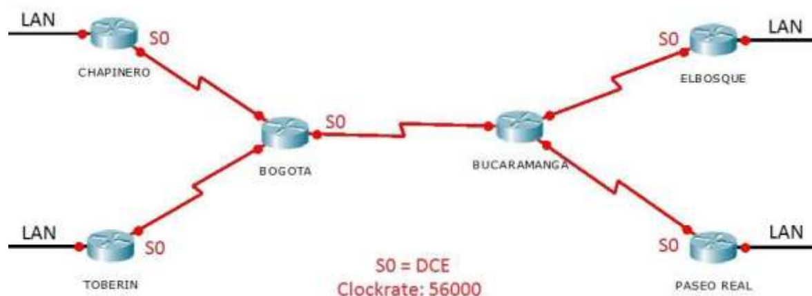
Figura 1. Topología física de la Red Pollosan
