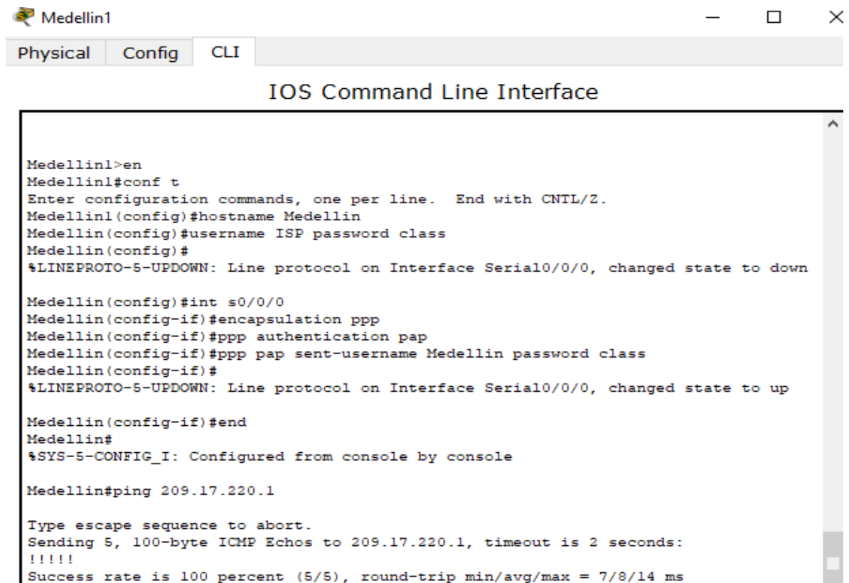
Ilustración 22. Se realiza ping de Medellin1 al ISP
