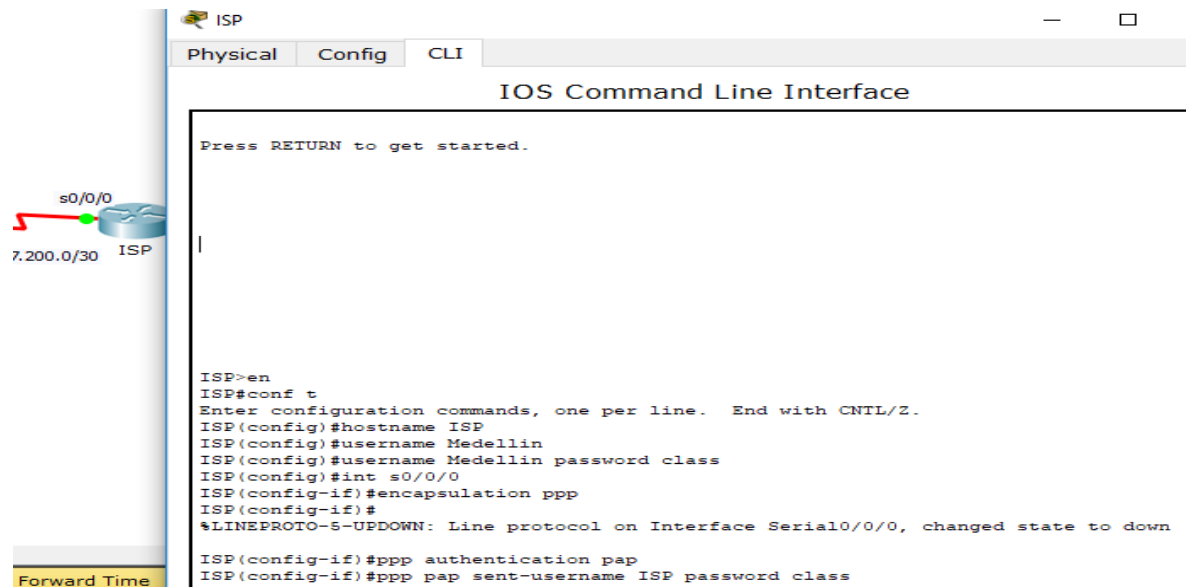
Ilustración 21. Autenticación con PAP
