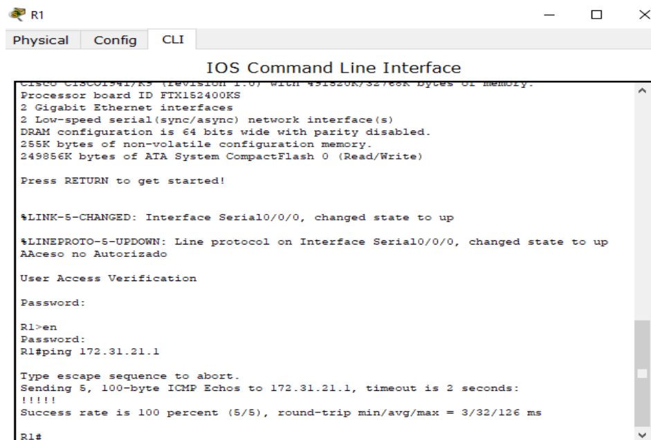
Ilustración 48. Ping de R1 al R2
