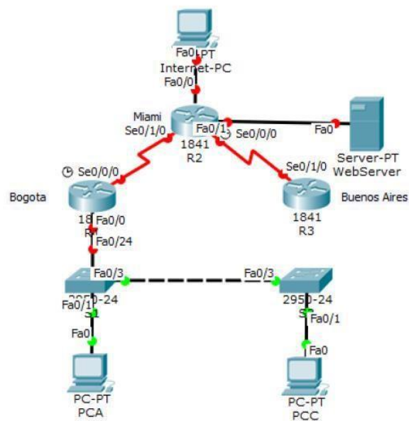
Ilustración 36. Topología Planteada Packet Tracer
