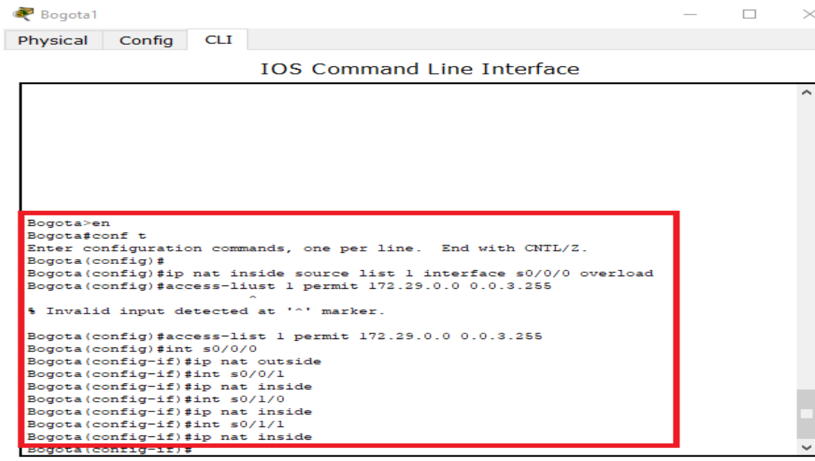
Ilustración 27. Indica las interfaces de entrada y salida Bogota1
