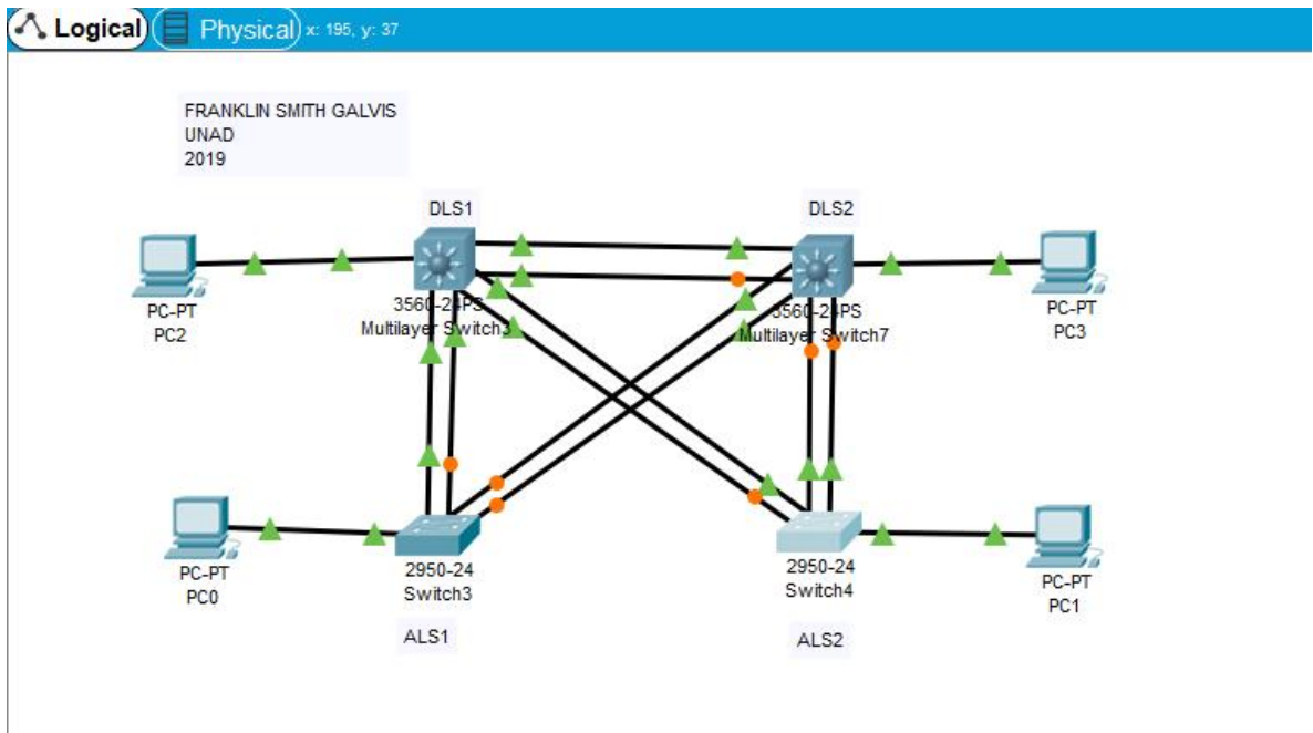
Ilustración 24. Topología Packet Tracer escenario-2- franklin Galvis
