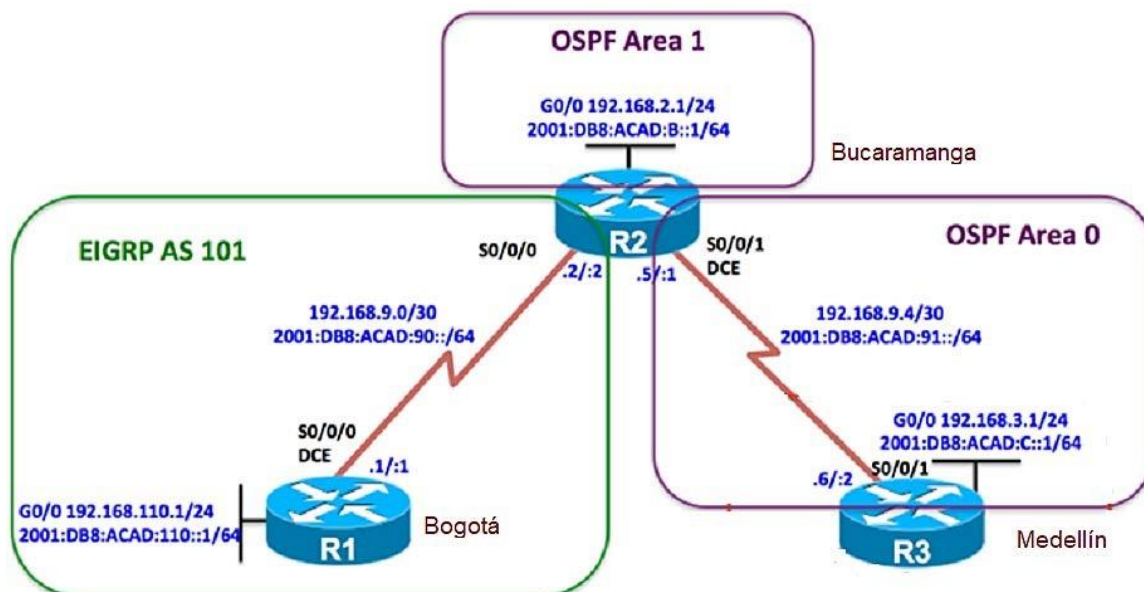
Figura 1. Topología escenario 1
