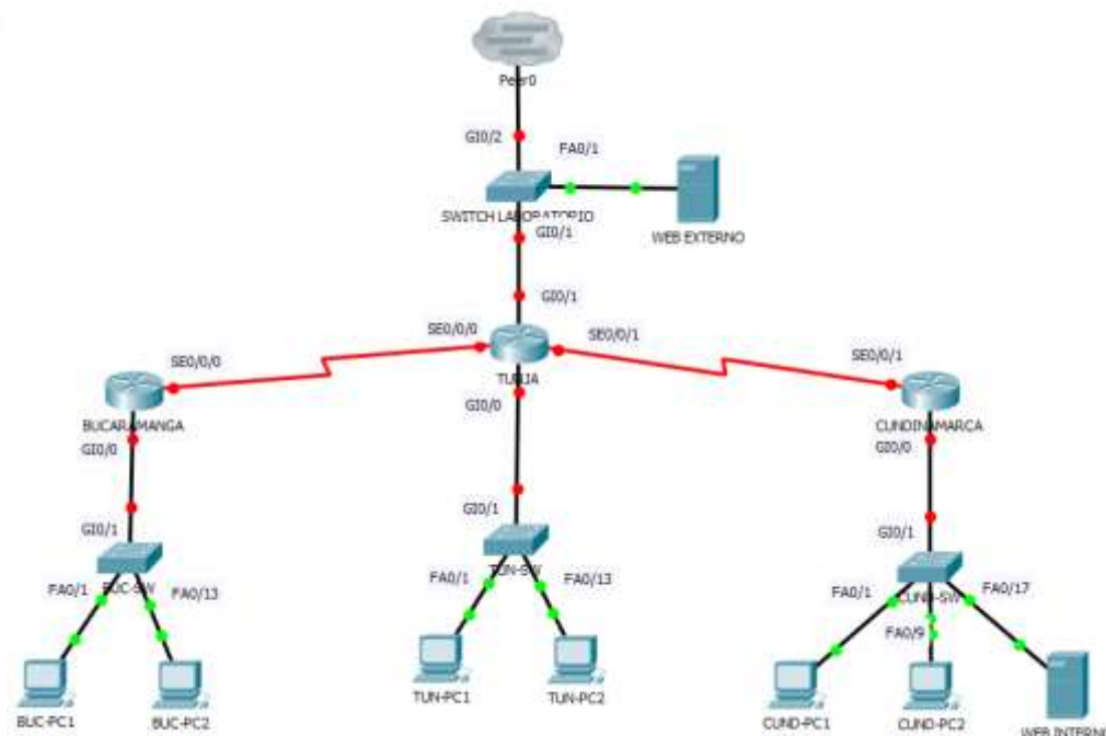
Ilustración 5. Topología - escenario 2
