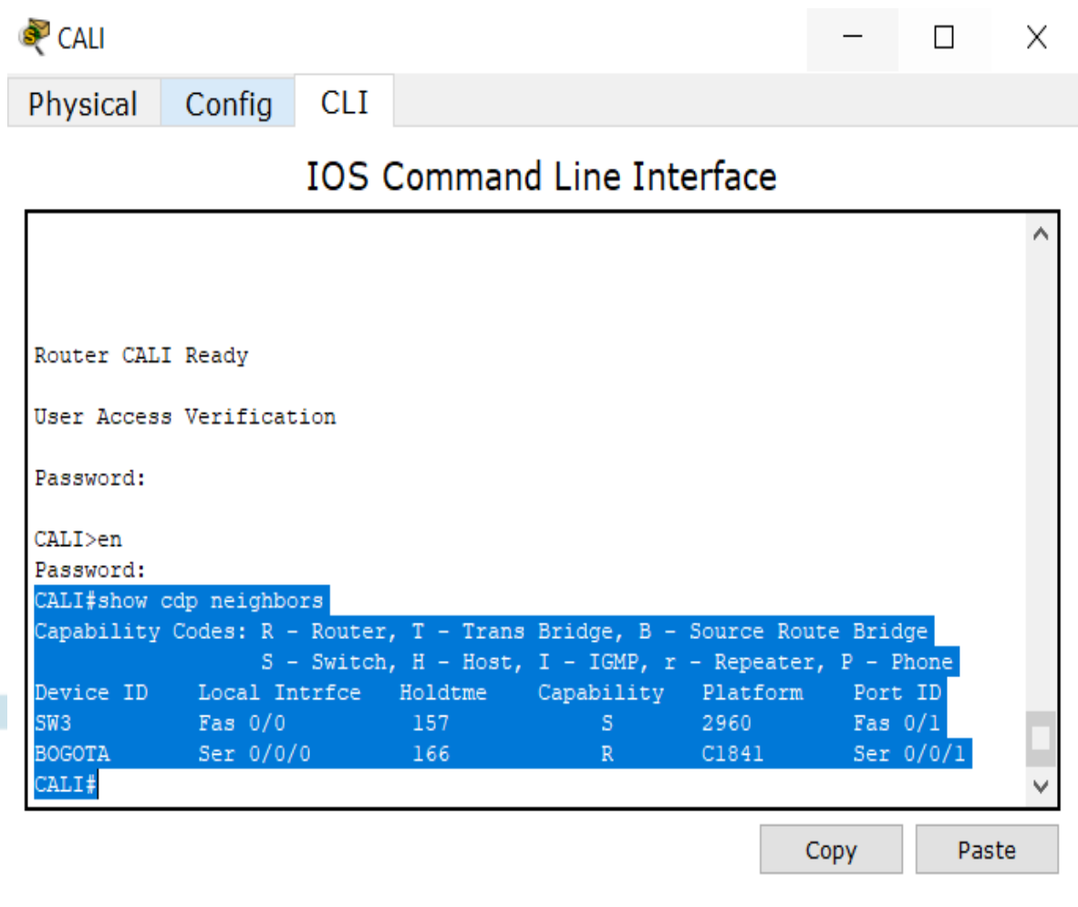
Gráfico 9. Gráfico 8. Comando "show cdp neighbors" en el Router "CALI" – Escenario 1
