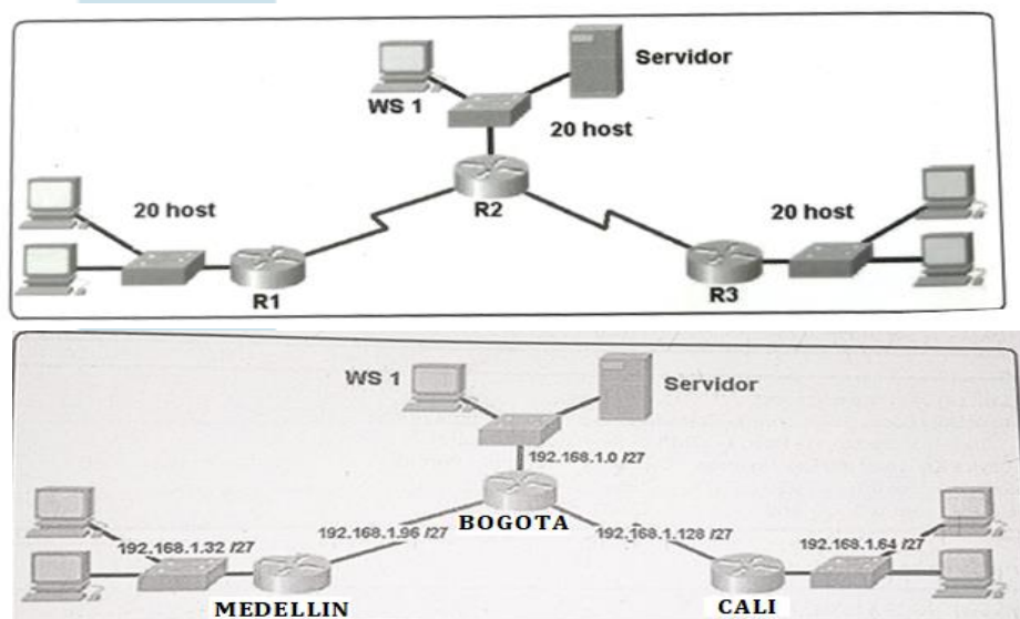
Gráfico 1. Topología de la Red Escenario 1
