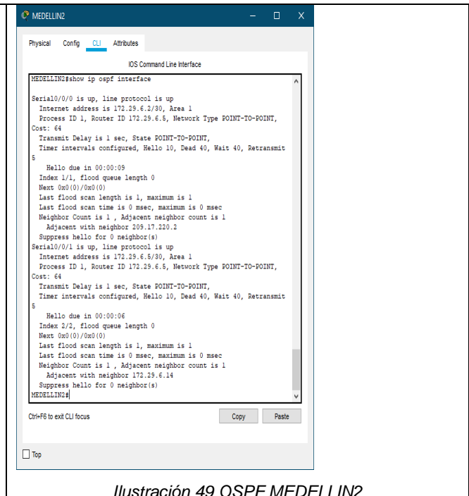
Ilustración 49 OSPF MEDELLIN2
