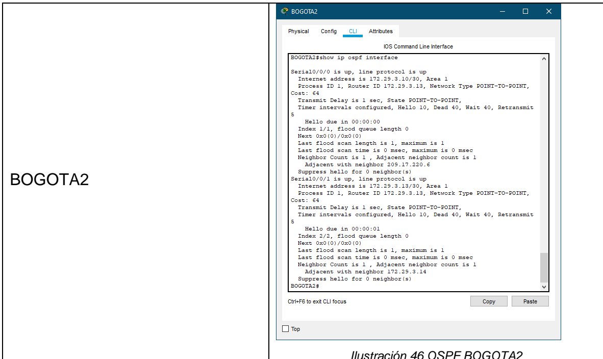
Ilustración 46 OSPF BOGOTA2
