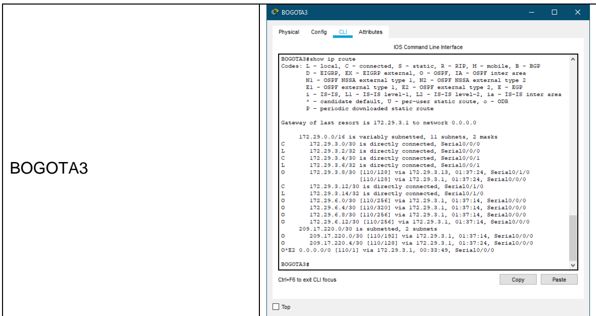
Ilustración 34 Rutas BOGOTA3
