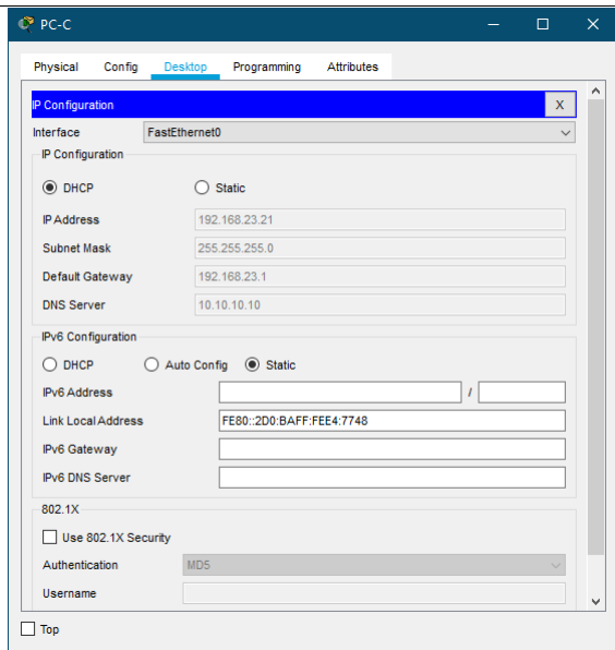
Ilustración 10 PC-C DHCP
