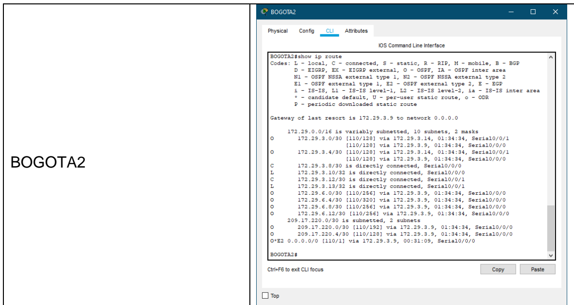
Ilustración 32 OSPF BOGOTA2
