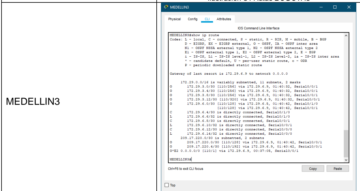
Ilustración 35 Rutas MEDELLIN3
