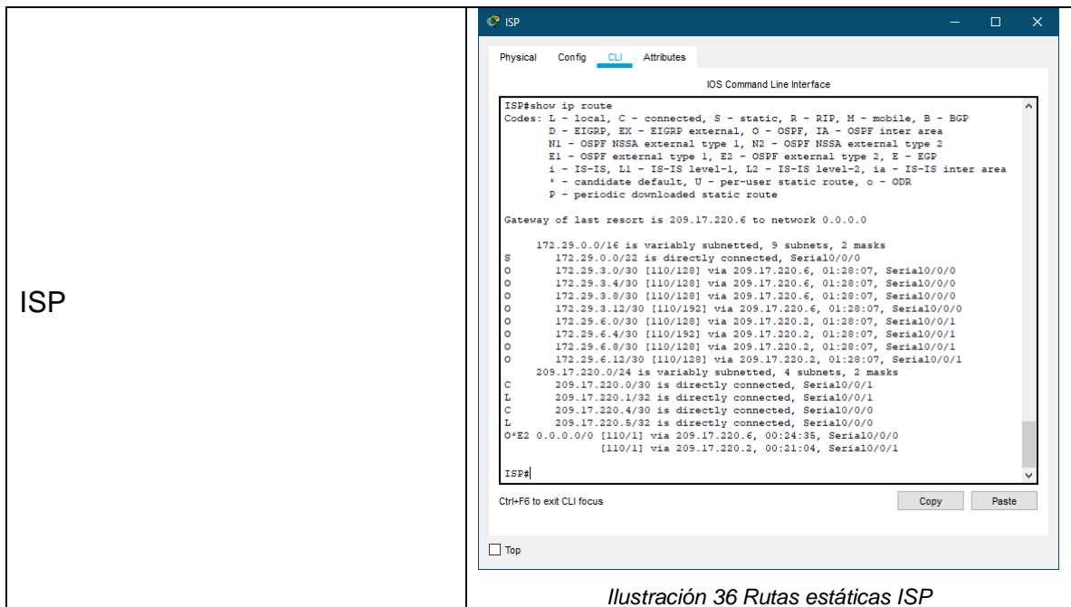
Ilustración 36 Rutas estáticas ISP
