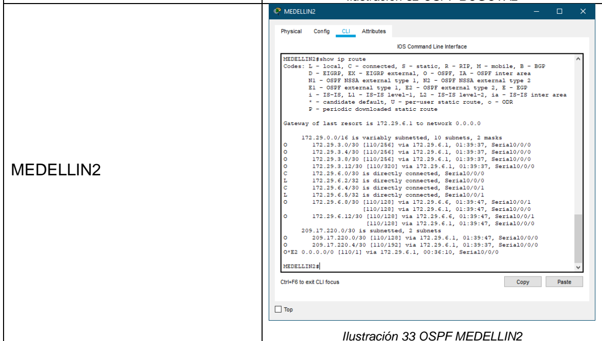
Ilustración 33 OSPF MEDELLIN2
