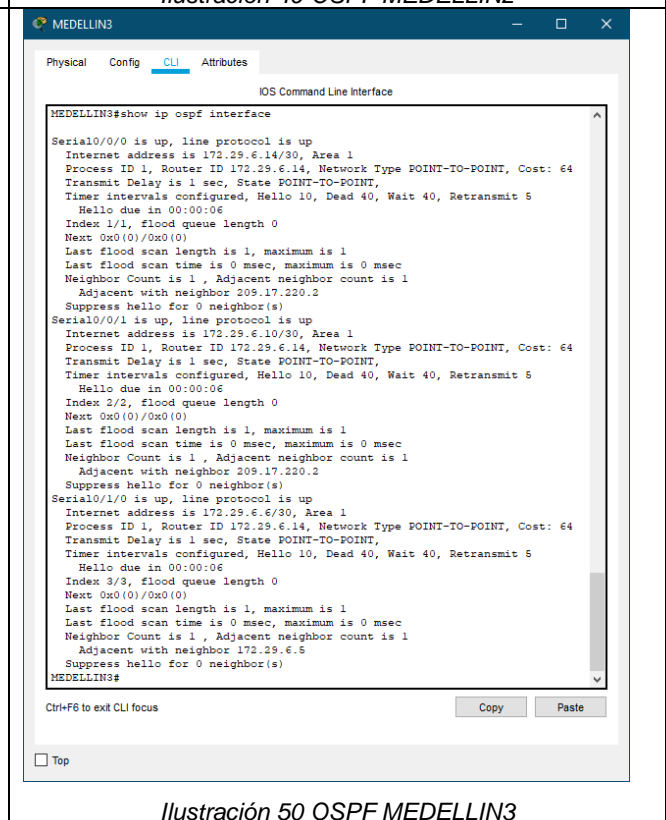
Ilustración 50 OSPF MEDELLIN3
