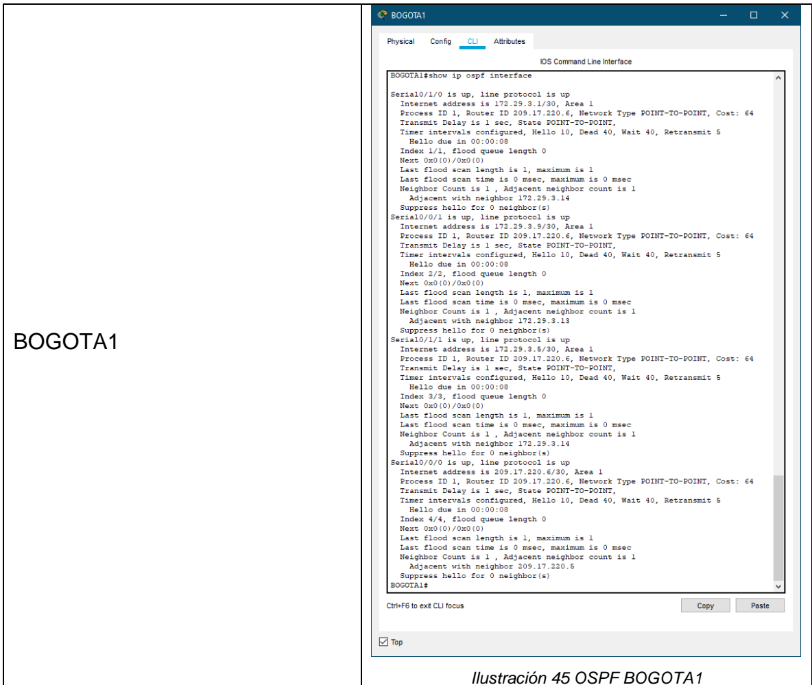
Ilustración 45 OSPF BOGOTA1
