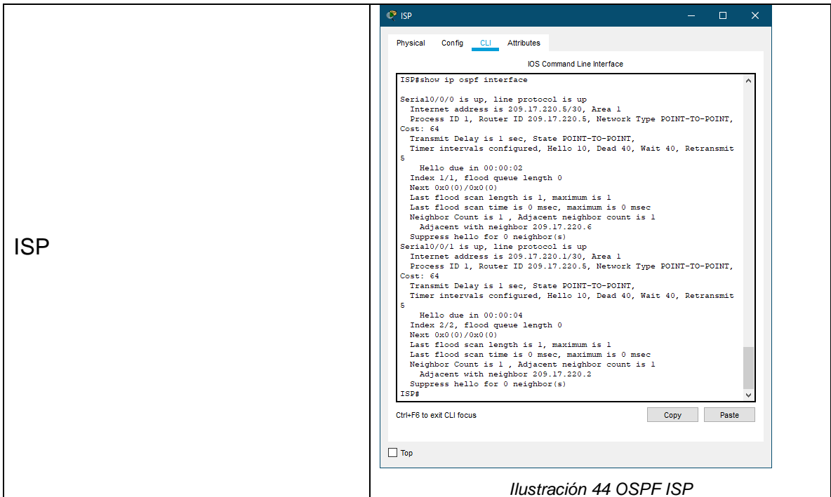
Ilustración 44 OSPF ISP
