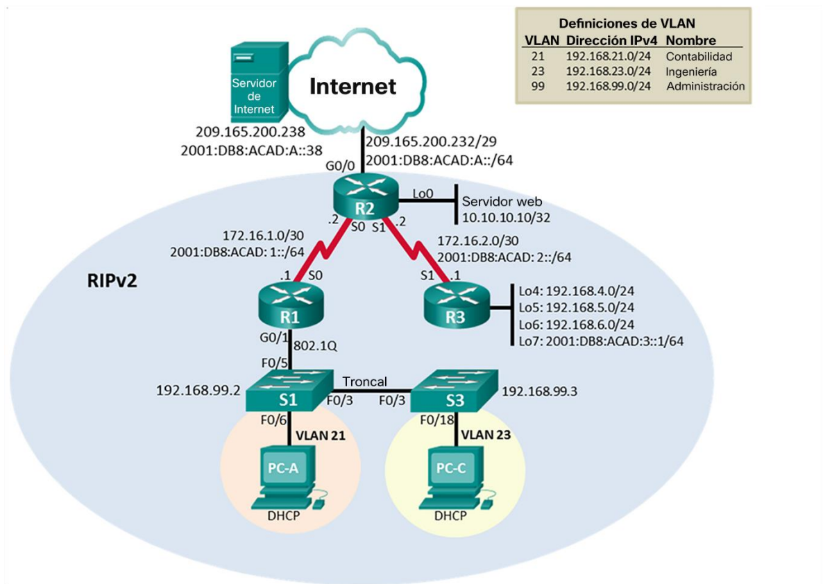
Ilustración 1 Topología de escenario 1
