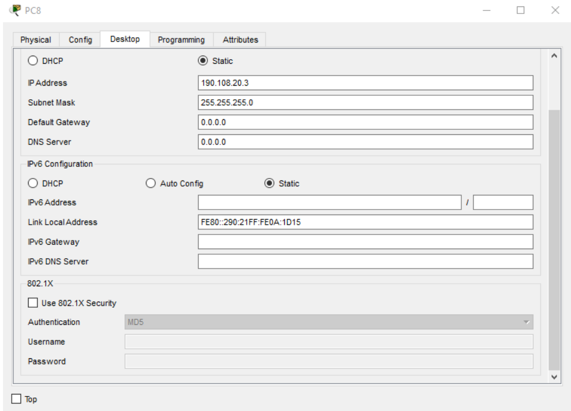
Figura 38. Asignaciones de las direcciones IP a los PCs
