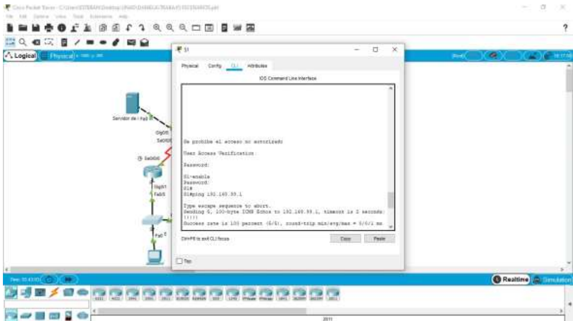
Figuras 5. Ping del S1 a la VLAN 99
