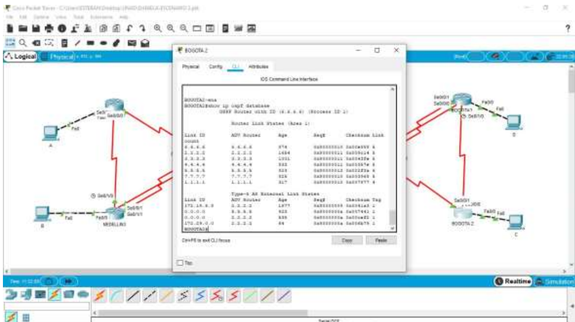
Figuras 33. Base de datos OSPF en BOGOTA2
