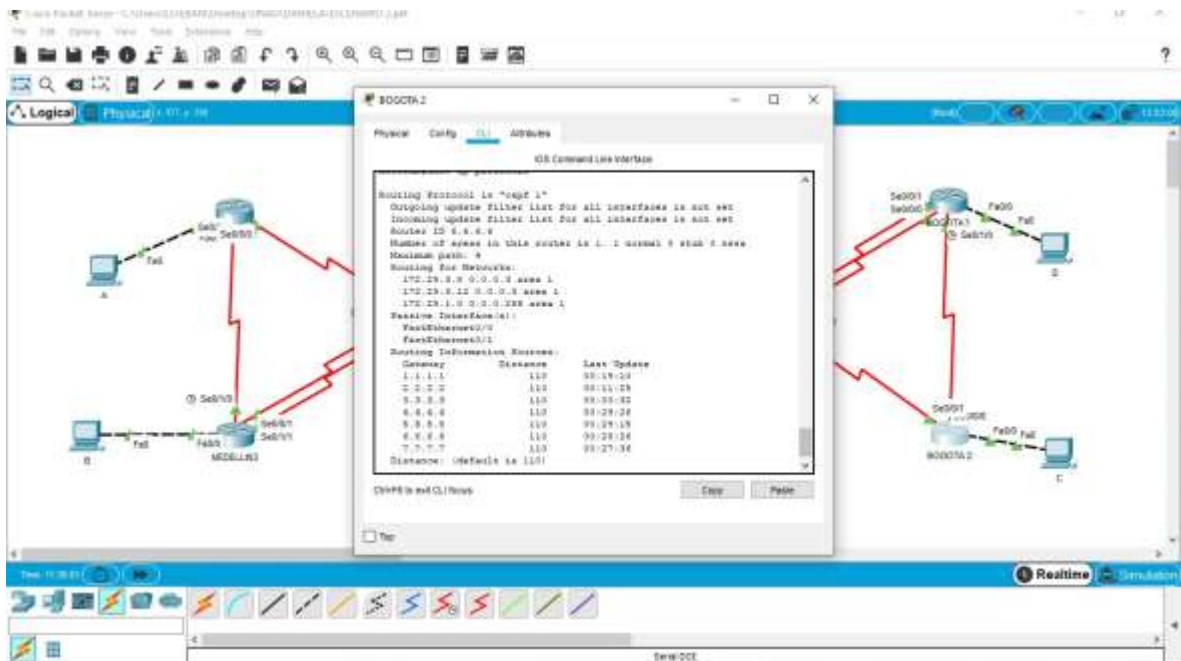
Figuras 32. Opciones de enrutamiento en BOGOTA2
