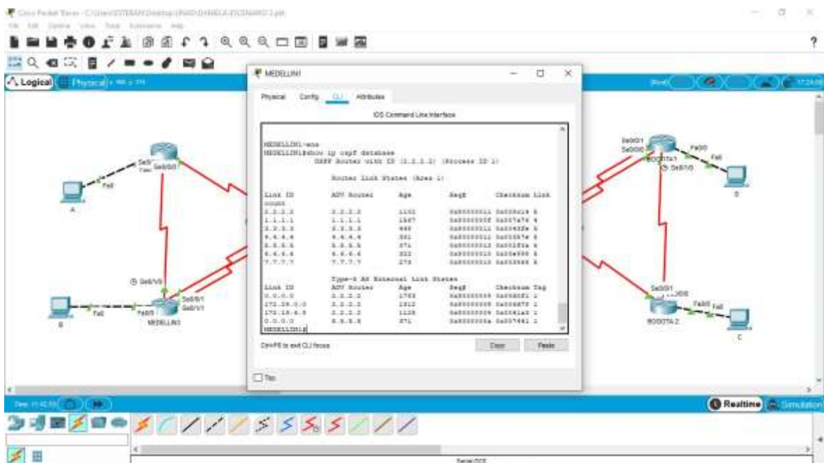
Figuras 25. Base de datos OSPF en MEDELLIN1
