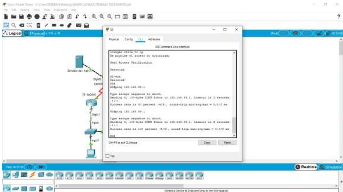
Figuras 6. Ping del S3 a la VLAN 99
