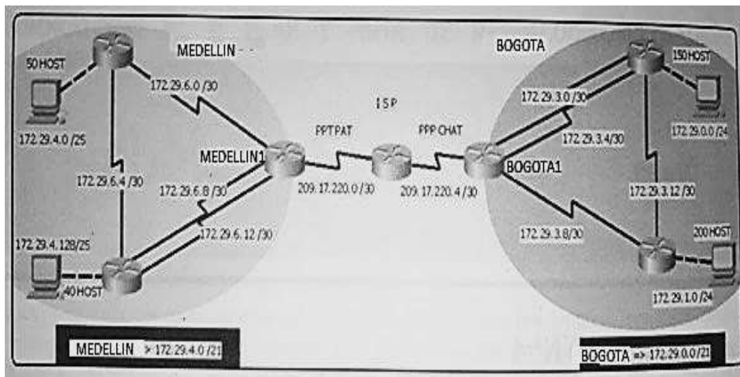
Figura19 topologia escenario 2
