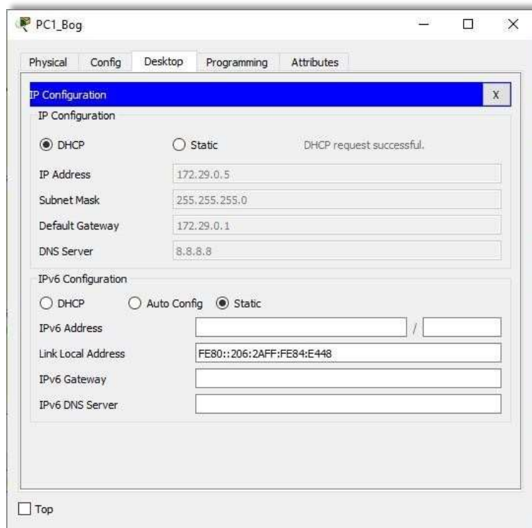
Figura 45. Configuración IP PC1_Bog.
