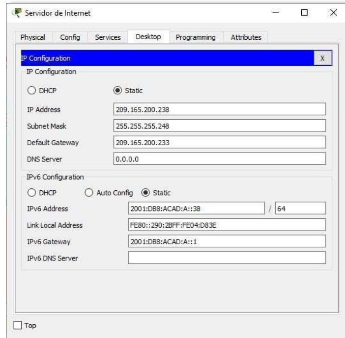
Figura 2. Configuración IP del servidor
