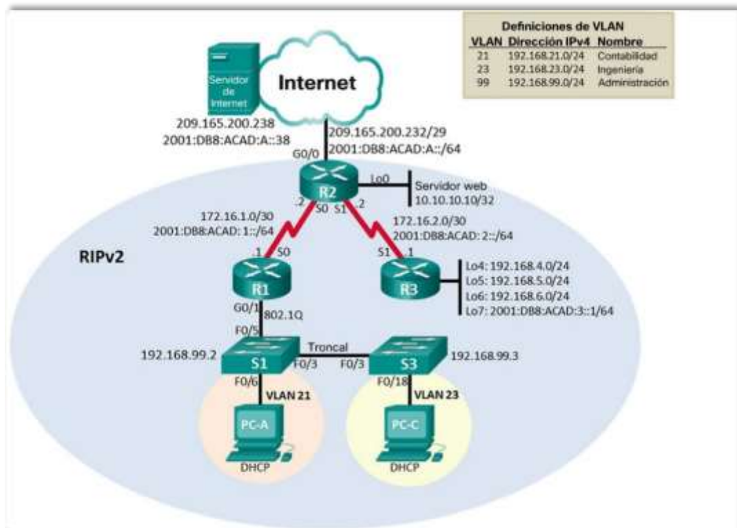
Figura 1. Topología de red escenario 1. 1
