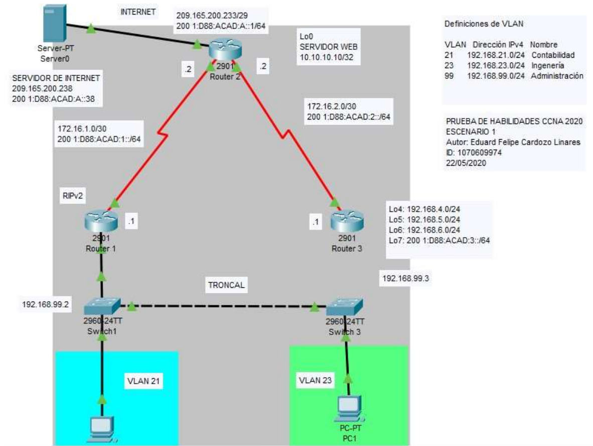
Figura 25. Topología de red del escenario – Cisco Packet Tracer.
