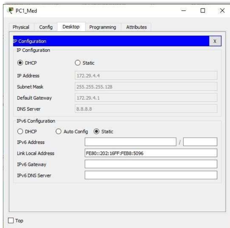
Figura 43. Configuración IP PC1_Med.
