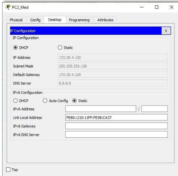
Figura 44. Configuración IP PC2_Med.
