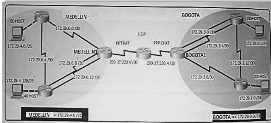
Figura 26. Topología de red escenario 2.
