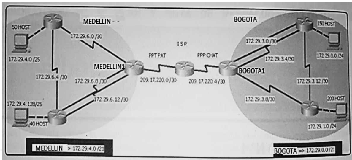
Figura 20. Topología de red escenario 2.
