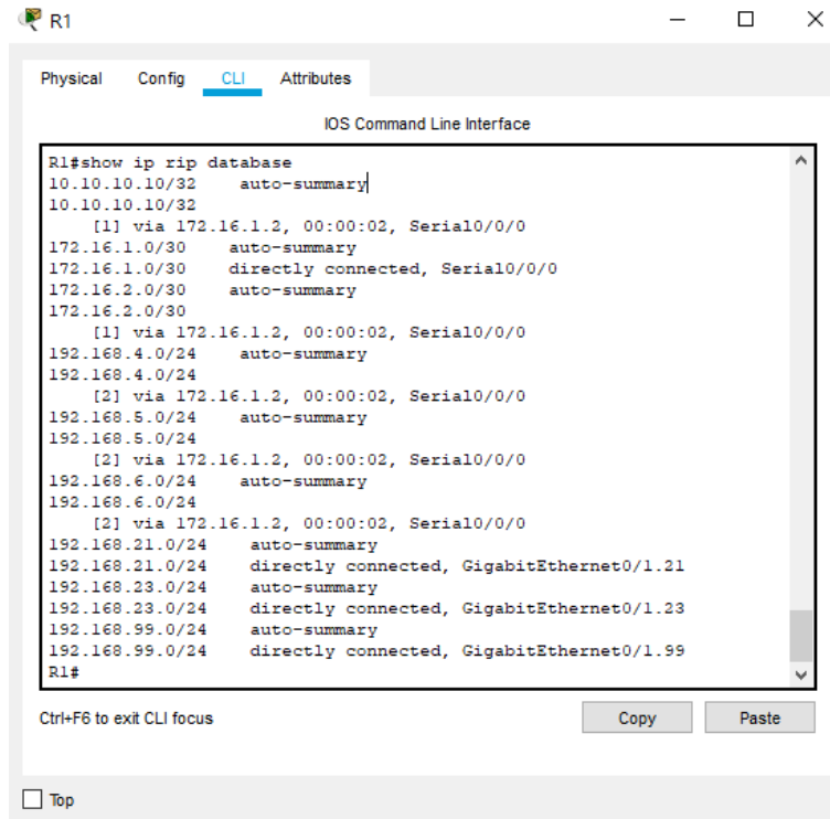
Figura 11. Se muestra la sección de RIP de la configuración en ejecución.
