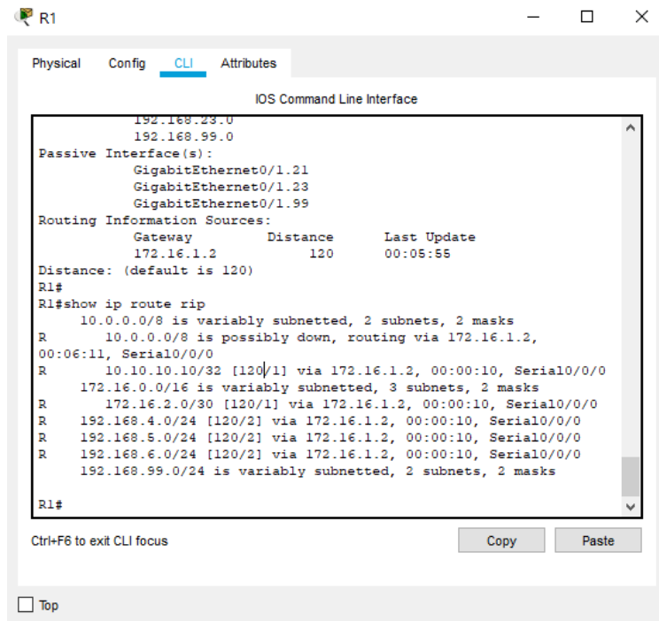
Figura 10. Se muestra solo las rutas RIP.
