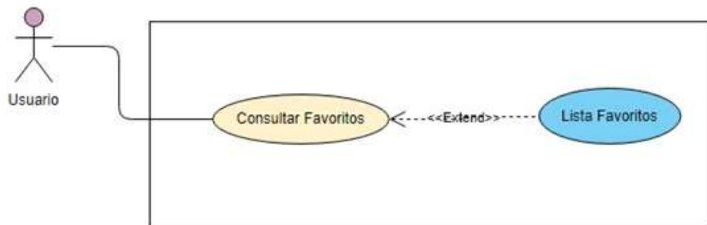
Figura 10. Caso de uso: Listar favorito - usuario autenticado
