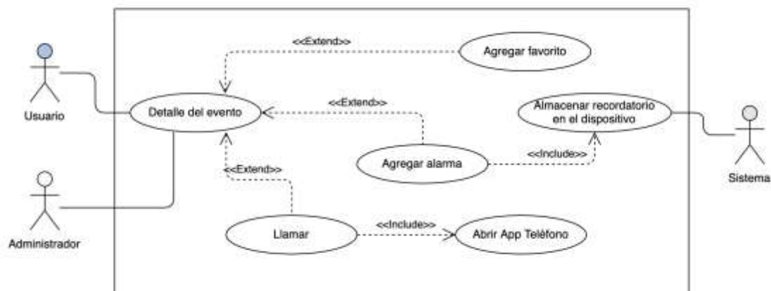
Figura 12. Caso de uso: Dashboard
