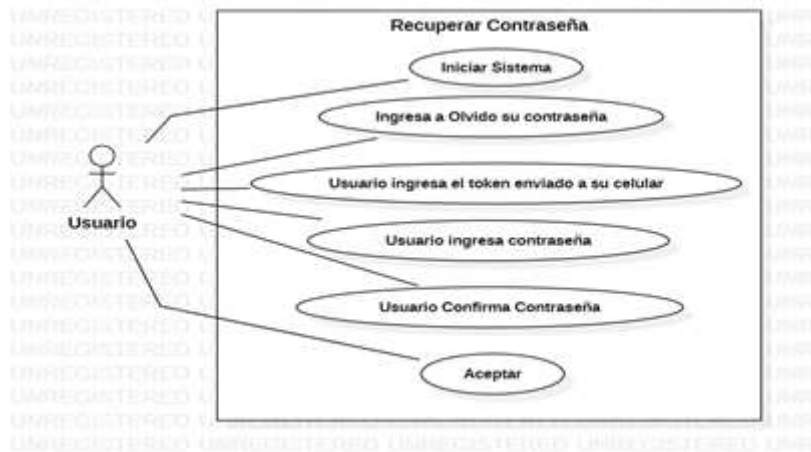
Figura 3. Caso de uso: Recuperar contraseña
