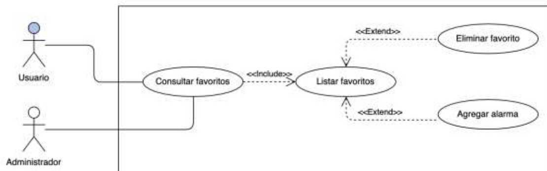
Figura 11. Caso de uso: Consultar favoritos
