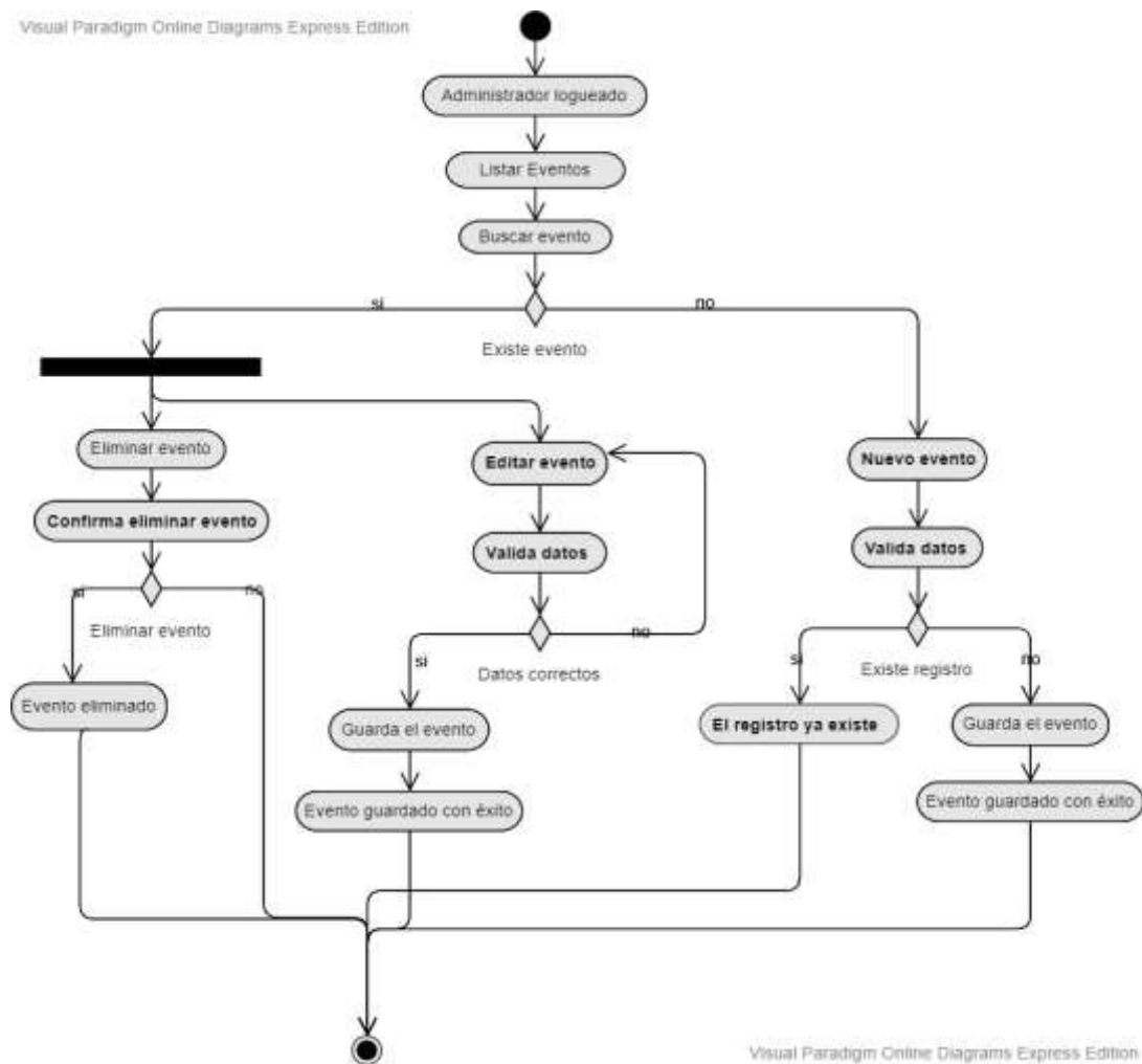
Figura 19. Diagrama de actividades: Administrar eventos
