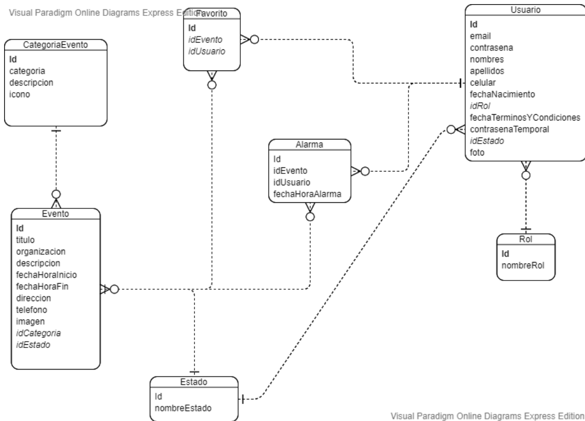
Figura 16. Modelo Entidad Relación
