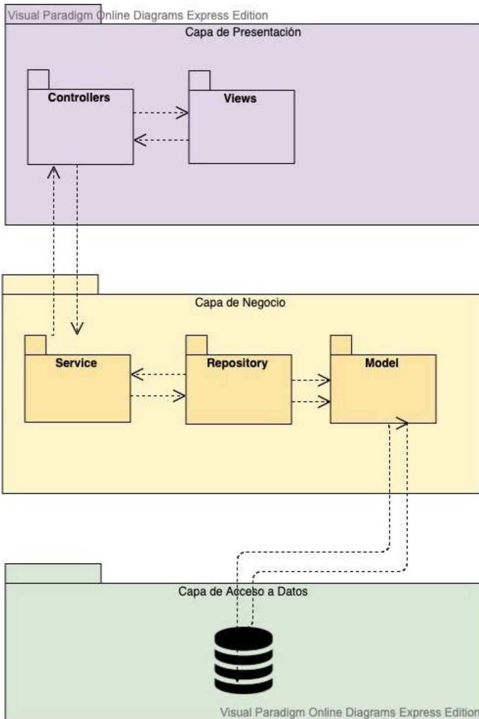
Figura 18. Diagrama de paquetes
