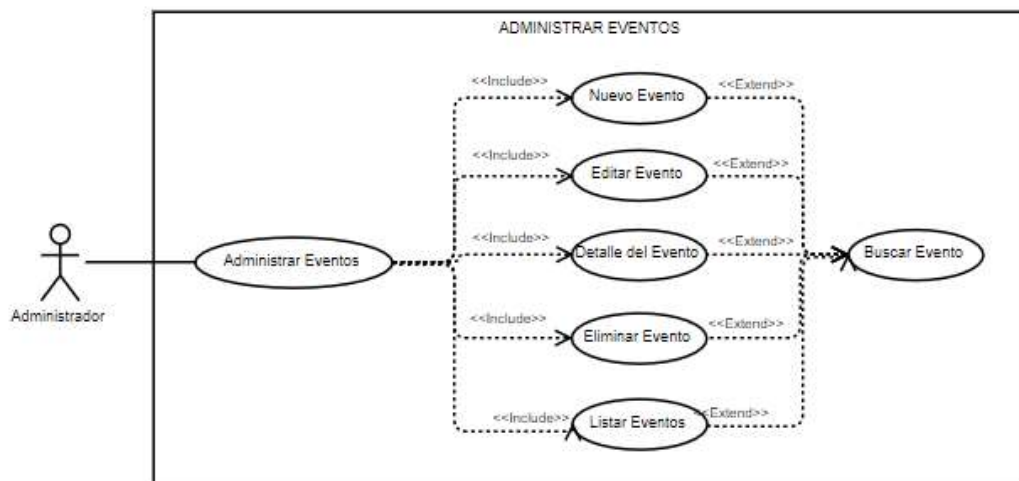
Figura 1. Caso de uso: Administrar eventos
