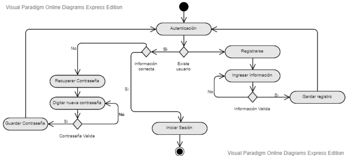
Figura 20. Diagrama de actividades: Autenticación
