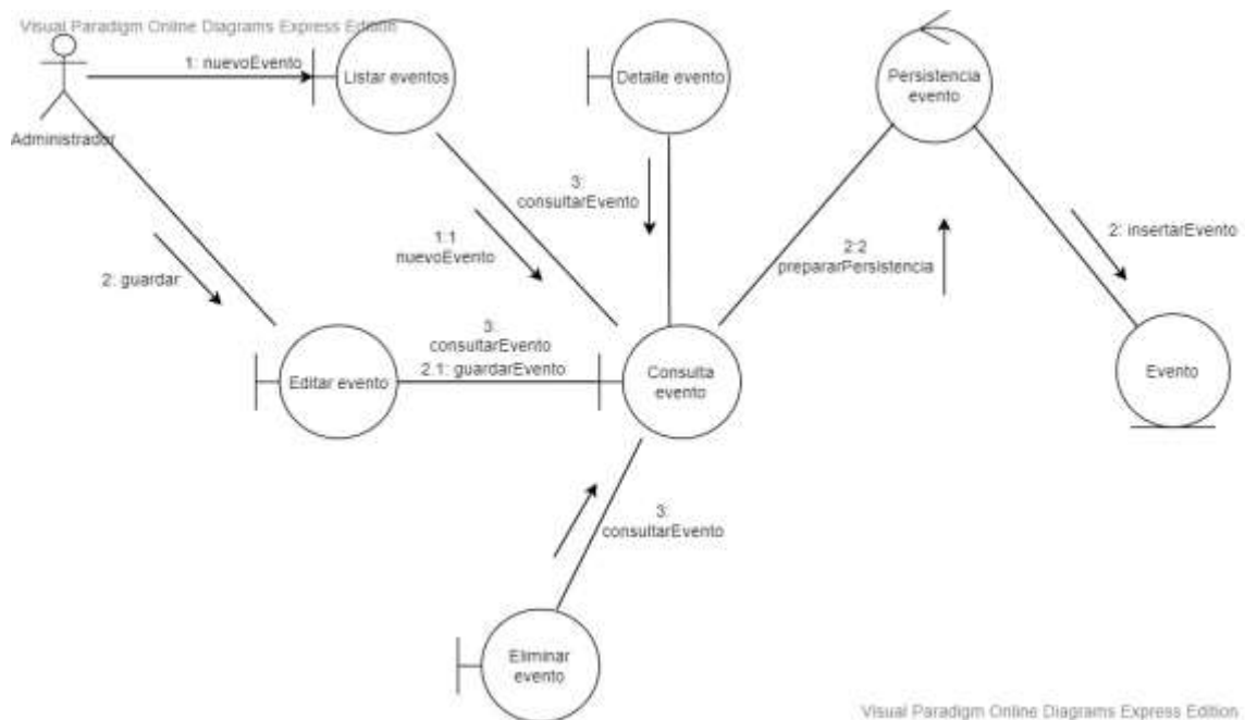
Figura 17. Diagrama de comunicación: Administrar eventos
