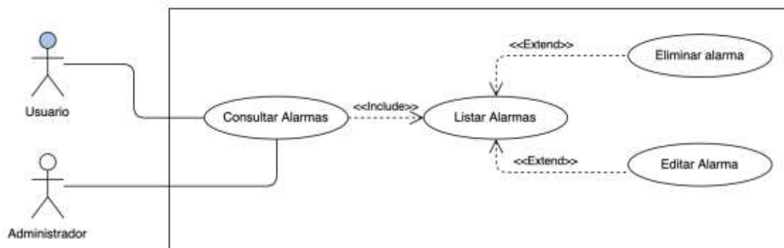
Figura 13. Caso de uso: Consultar alarmas
