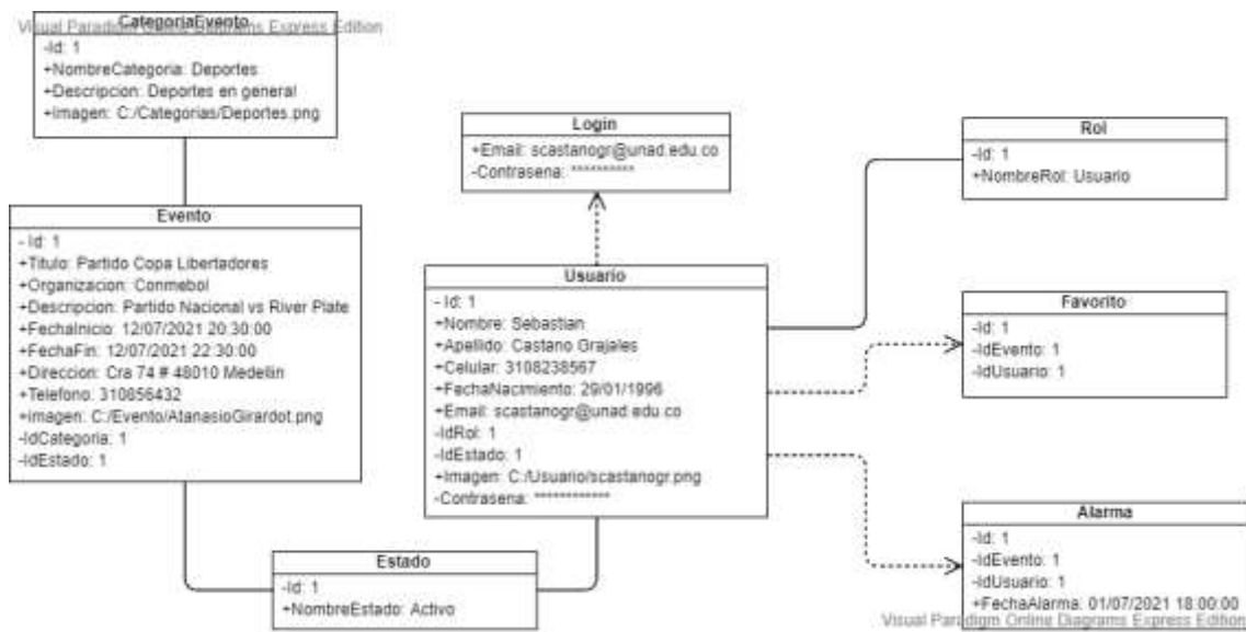
Figura 15. Diagrama de objetos
