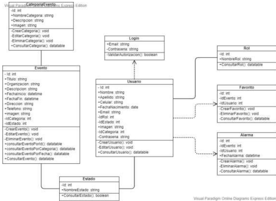
Figura 14. Diagrama de clases
