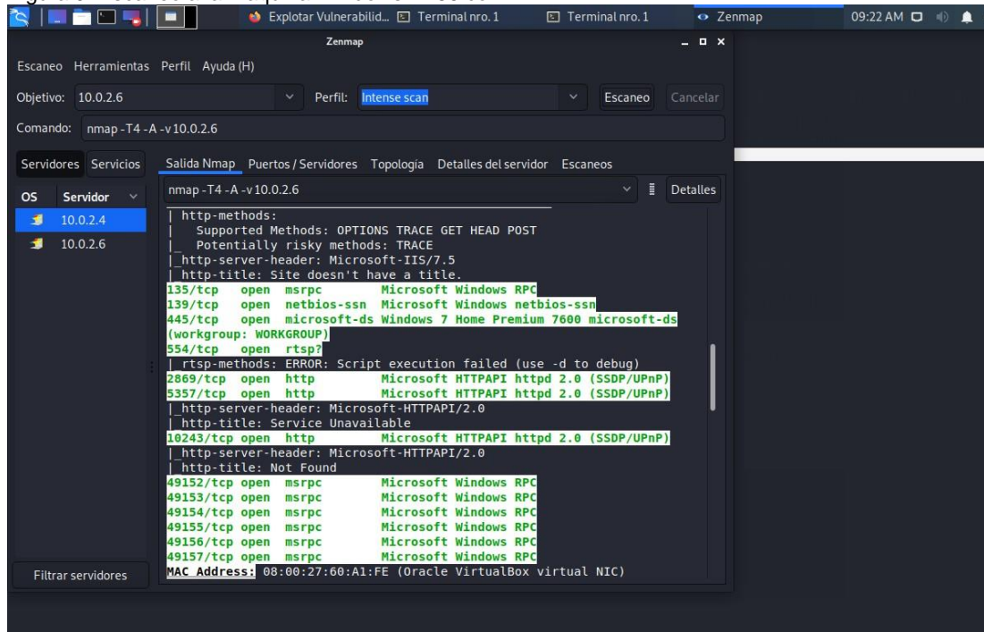
Figura 9. Escaneo a la maquina Windows 7X86 con ZENMAP
