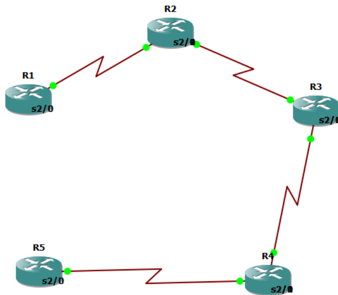
Figura 2. Conexión de Routers en GNS3
