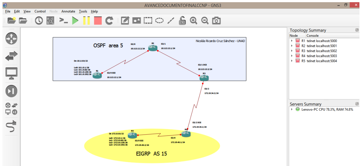
Figura 2. Topología primer escenario en GNS3
