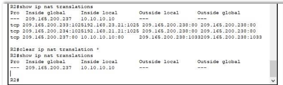
Figura 30 Eliminar las traducciones de NAT dinámicas.
