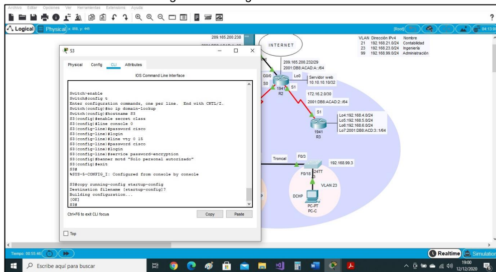
Figura 55. Configuración Switch 3
