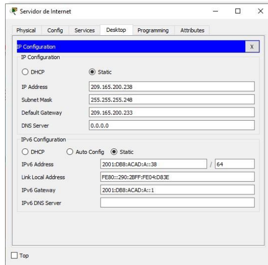
Figura 2. Configuración IP del servidor
