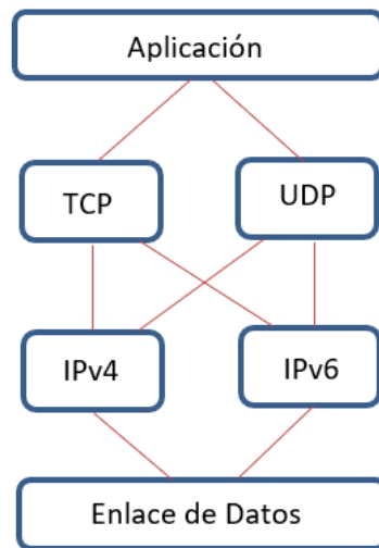
Figura 2. Mecanismo Dual Stack. (2020). Autor
