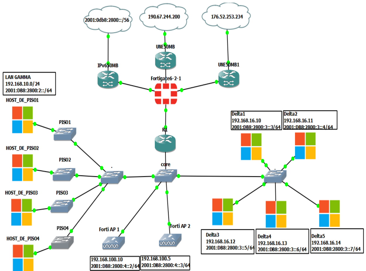
Figura 7. Diagrama de red en el protocolo IPv6 diagrama en Gns3. (2020). Autor
