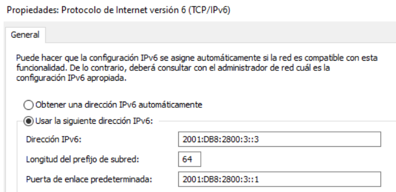
Figura 16. Direccionamiento IPv6 en host de red servidores. (2020). Fuente Autor.
