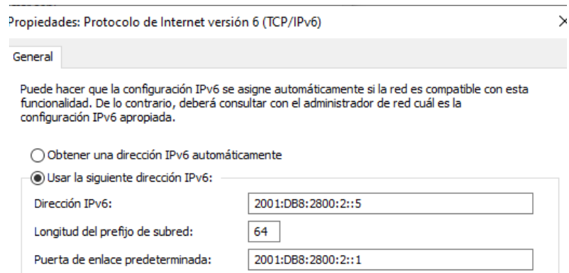
Figura 13. Direccionamiento IPv6 en host A en red LAN. (2020). Fuente Autor.
