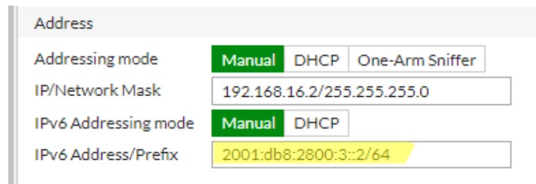
Figura 14. Asignación prefijo IPv6 en interfaz de firewall servidores. (2020). Fuente Autor.
