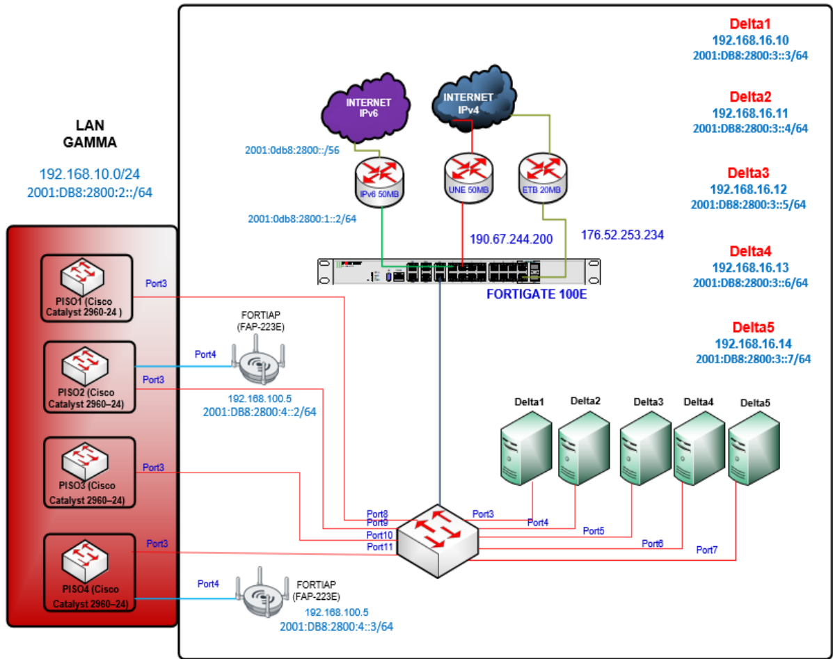
Figura 6. Diagrama de red en doble pila diagrama en Visio. (2020). Autor
