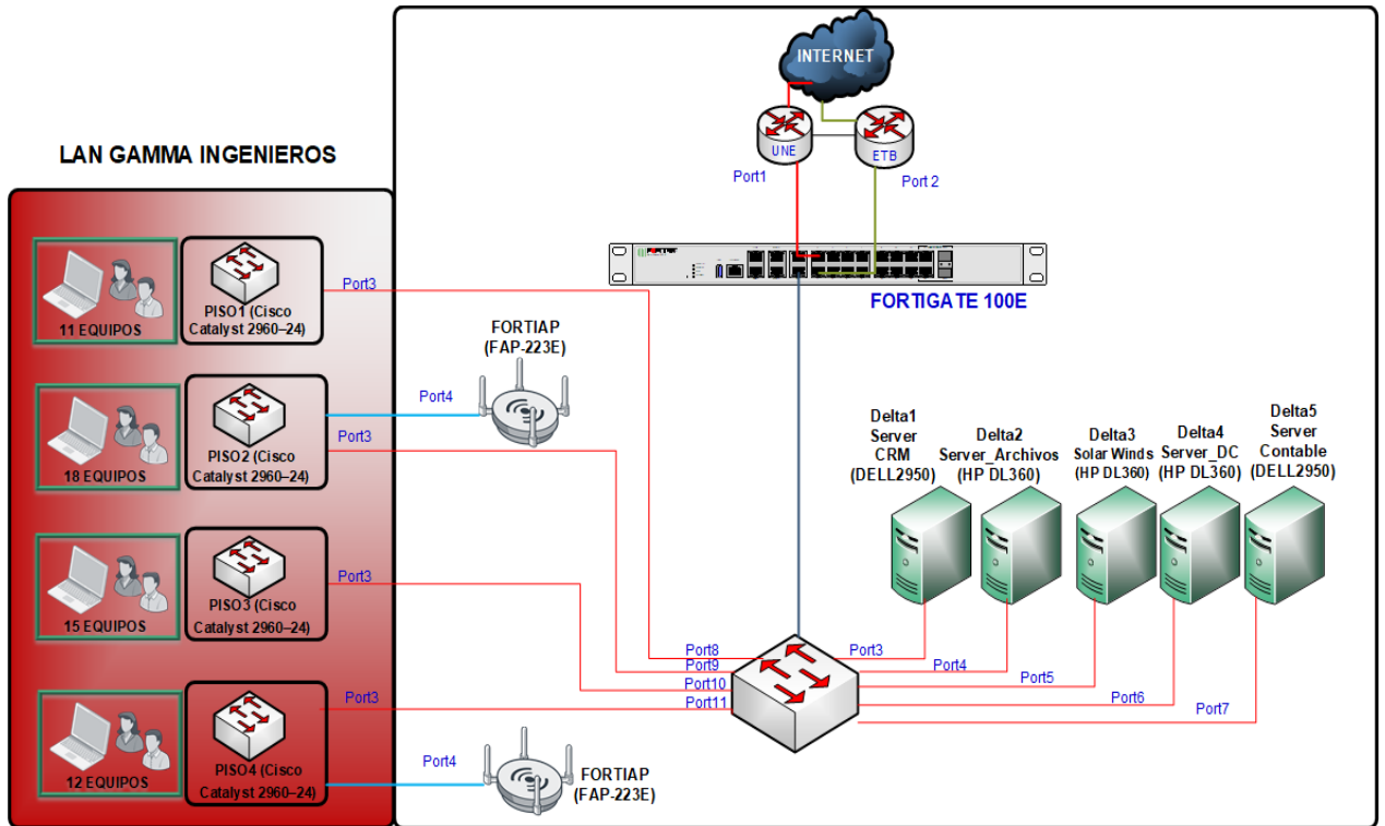
Figura 4. Topología de red Gamma Ingenieros diagrama en Visio. (2020). Autor
