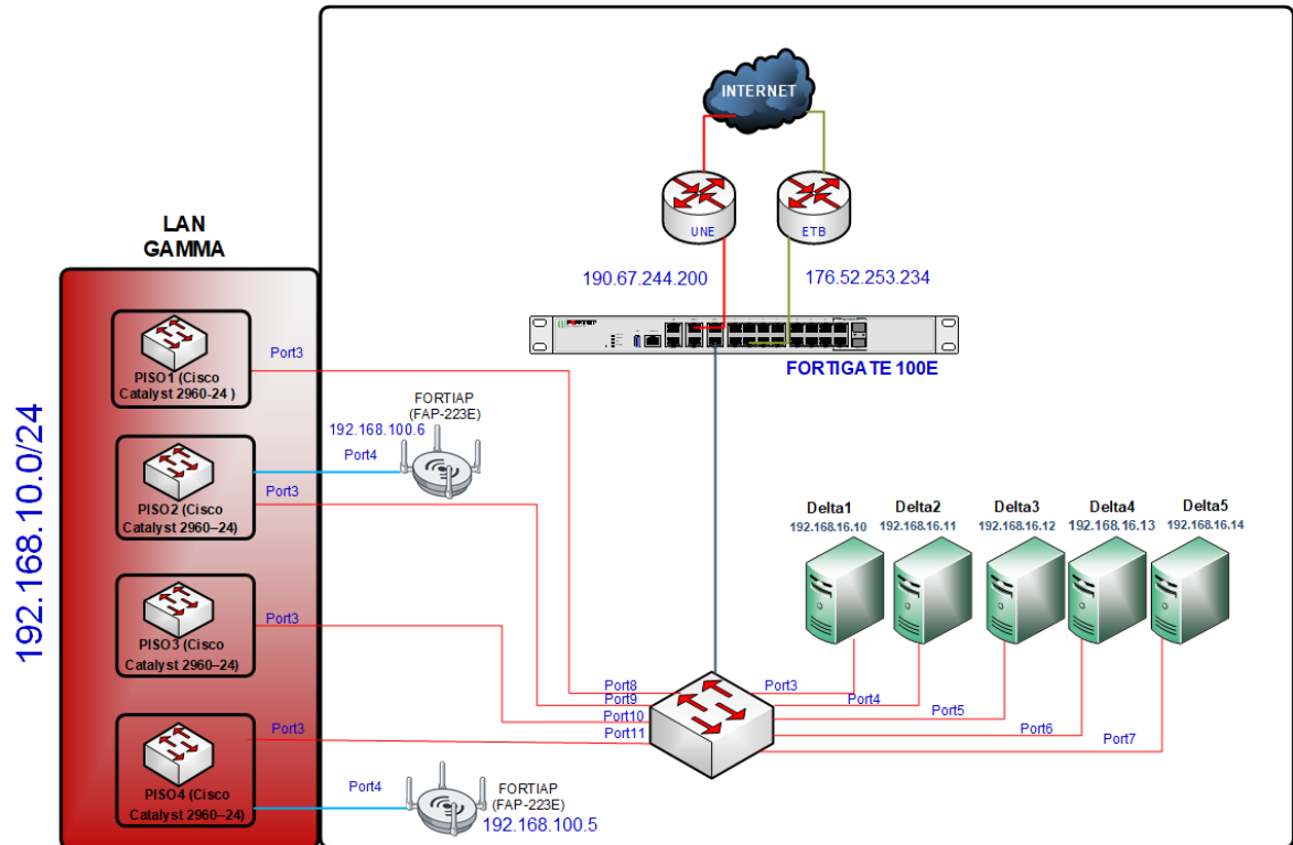
Figura 5. Direccionamiento IPv4 en red Gamma Ingenieros, diagrama en Visio. (2020). Autor
