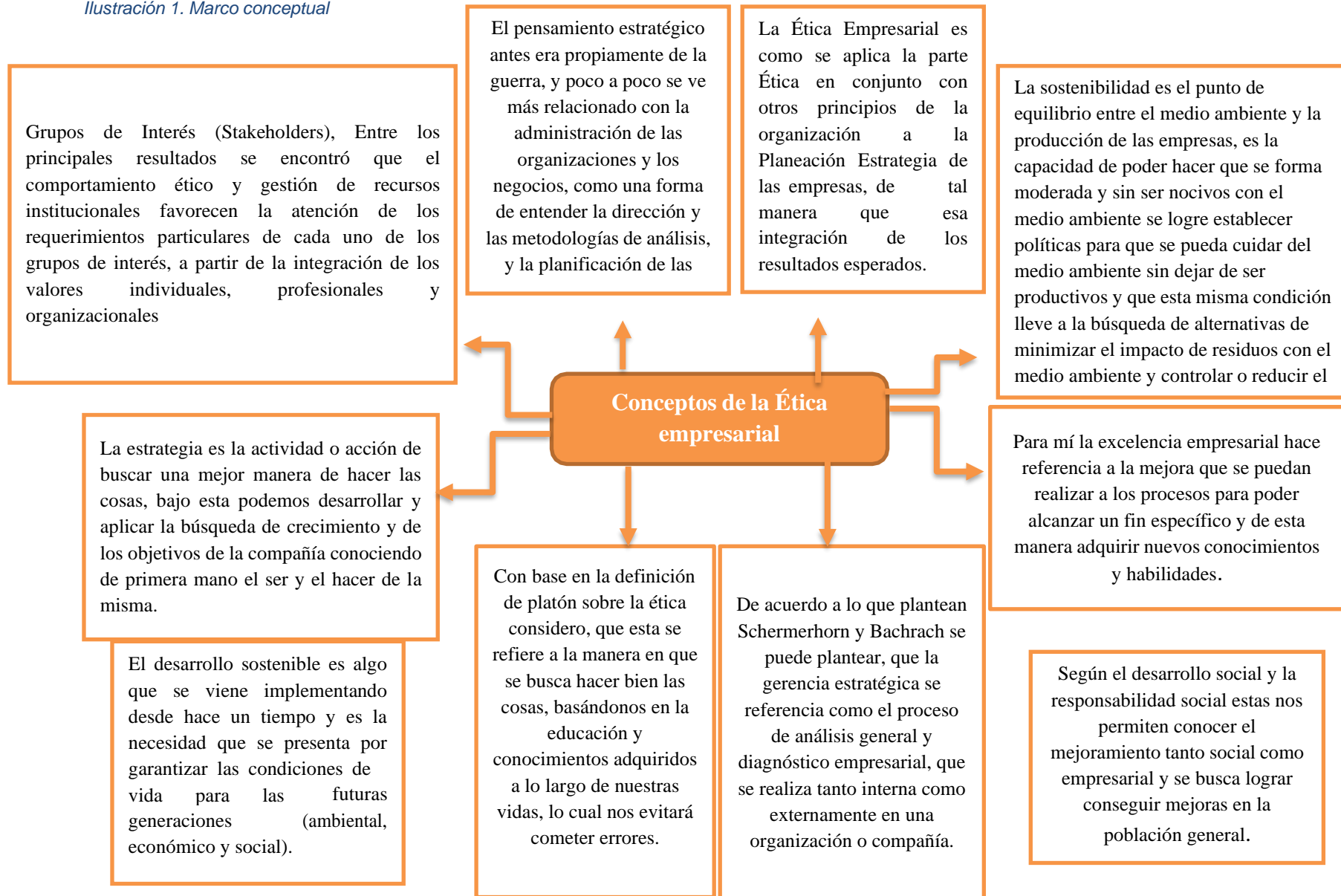
Ilustración 1. Marco conceptual
