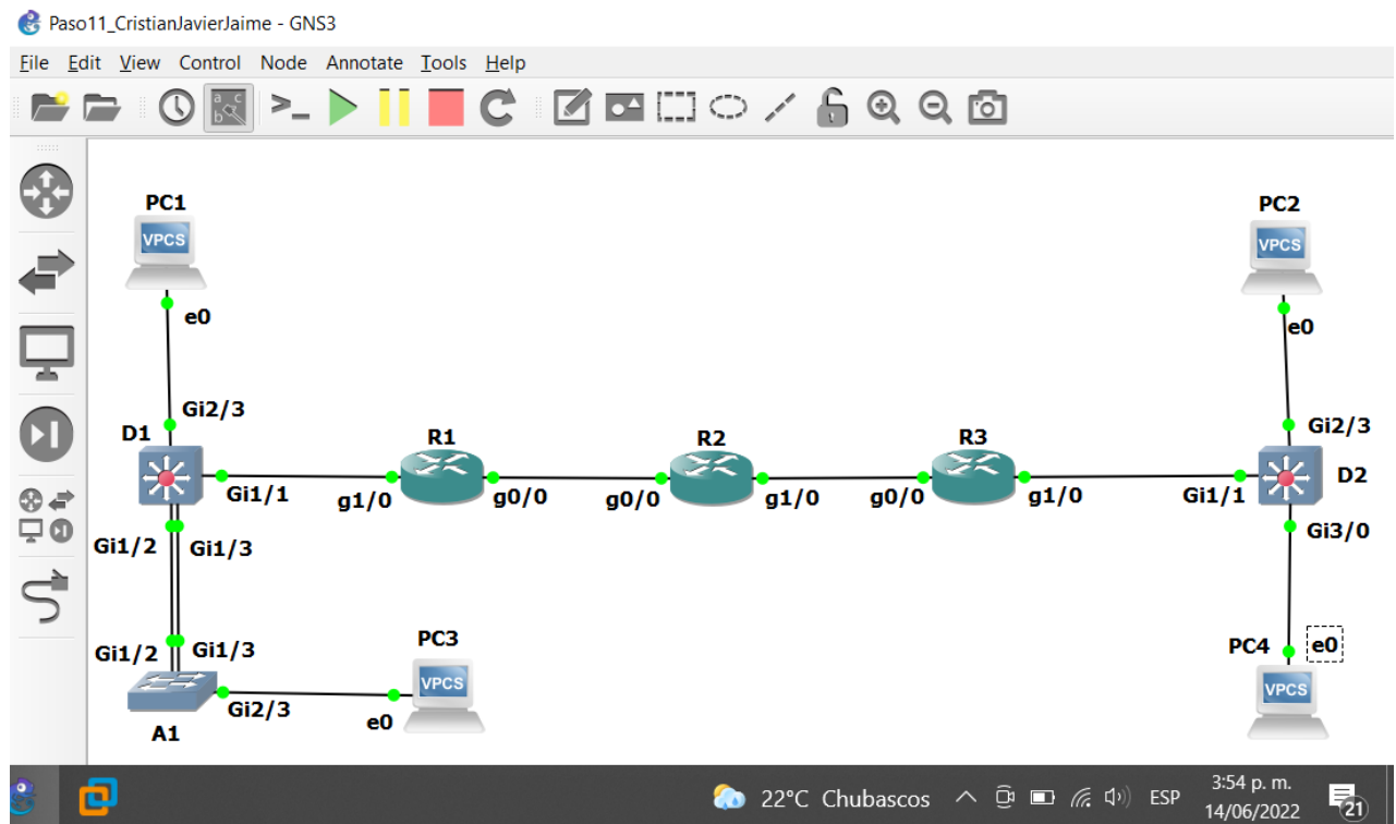
Figura 2. Implementación de la topología en GNS3. Fuente: Autor.
