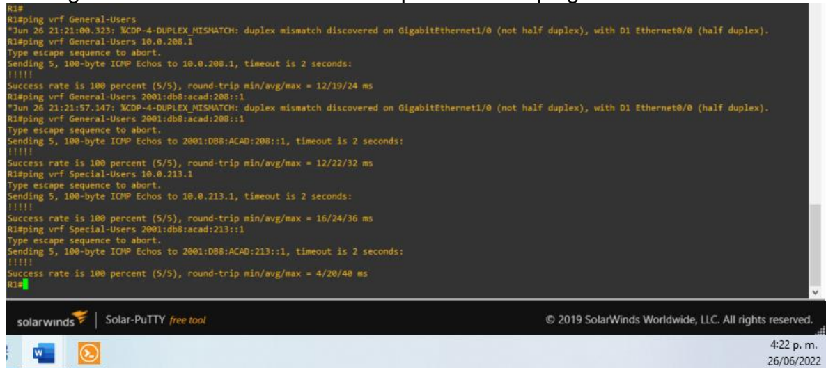
Figura 7. Verificación en cada VRF por medio de ping desde el Router R1.
