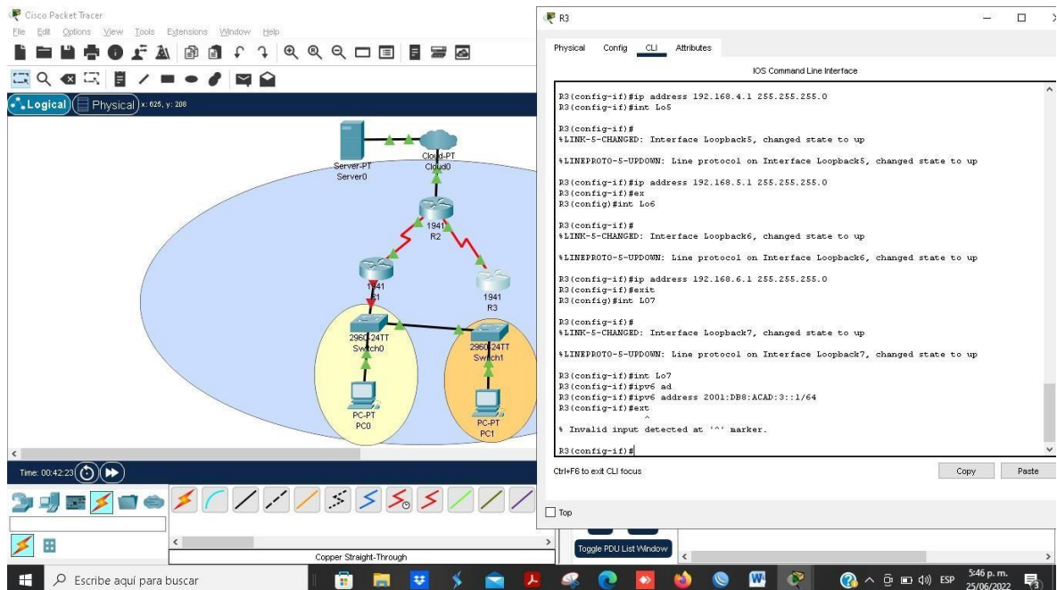
Figura 15. Configuración del router 3.
