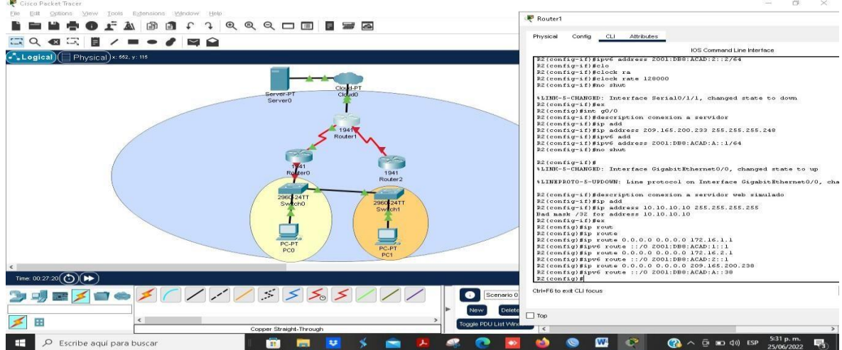
Figura 14. Configuración del router 2.
