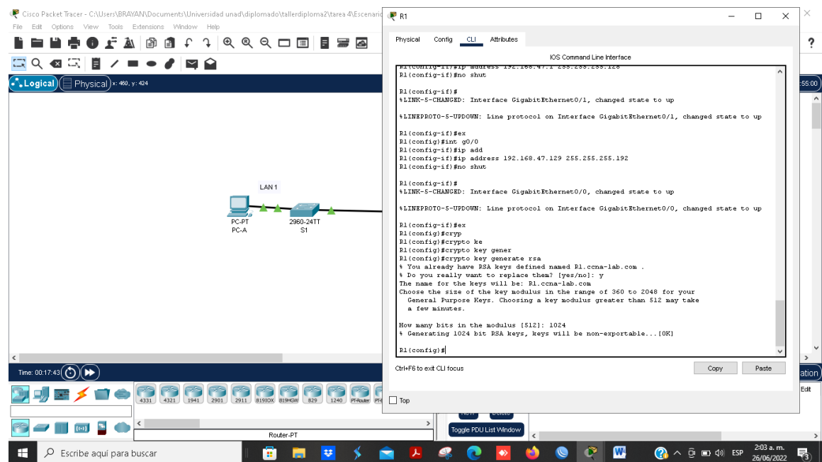
Figura 4. Guardado de configuración en la NVRAM.
