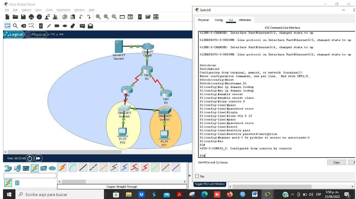
Figura 17. Configuración del switch 1.
