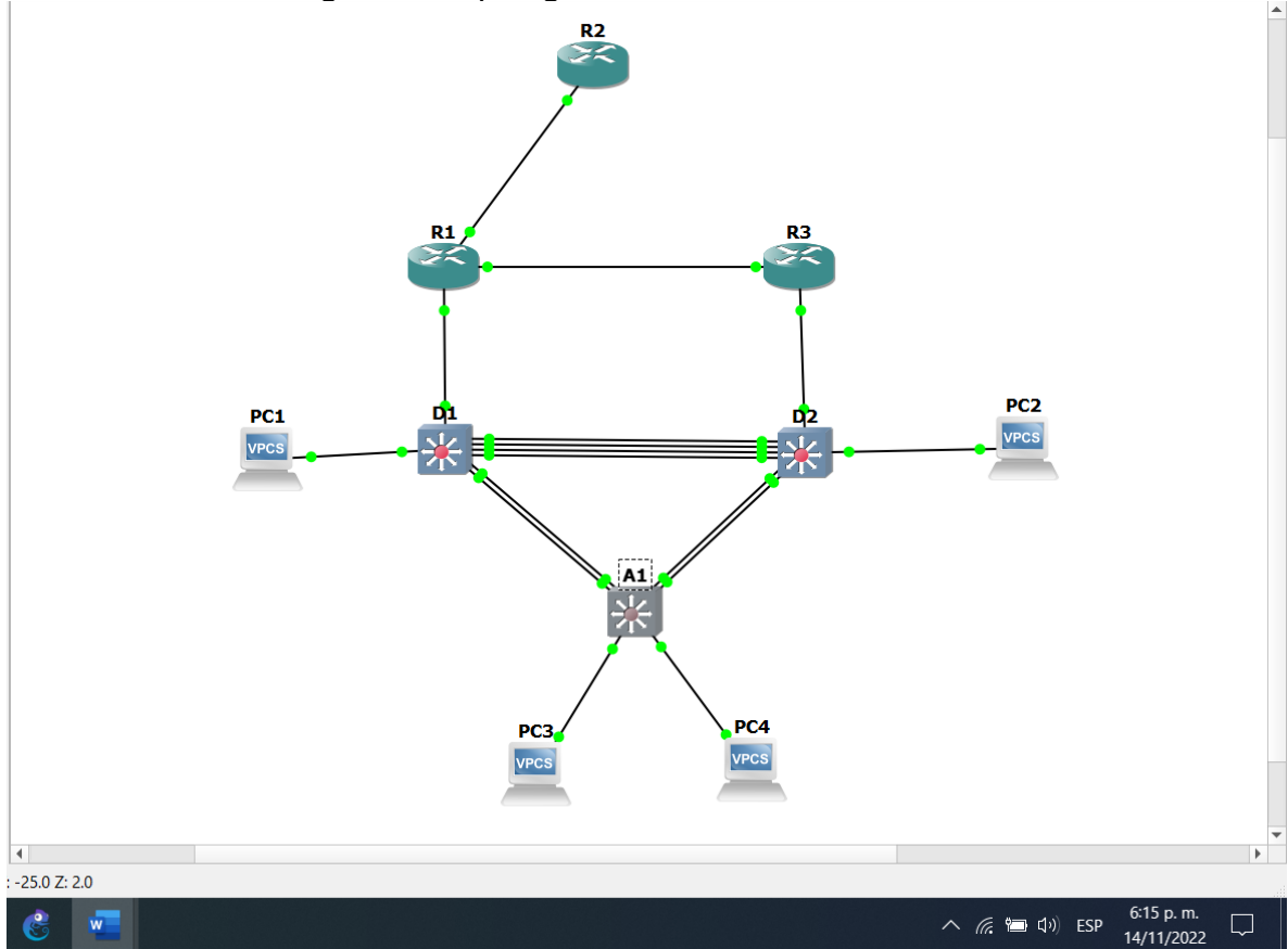
Figura 2. Topología del escenario 1 en GNS3.
