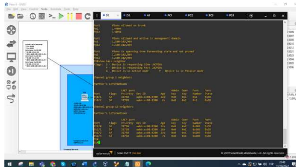
Figure 13. Comprobación de LACP Switch D1
