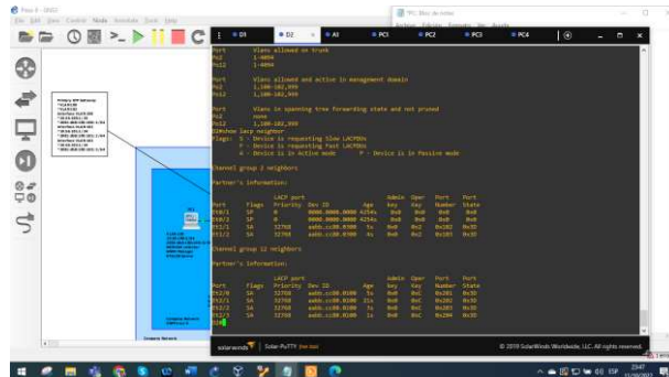
Figure 14. Comprobación de LACP Switch D2
