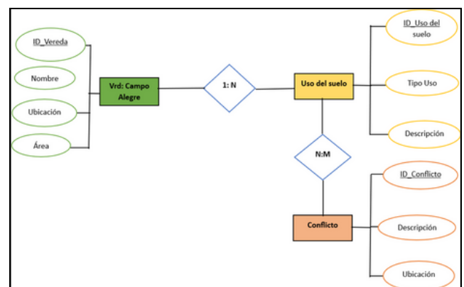
Figura 3: Modelo Entidad – Relación
