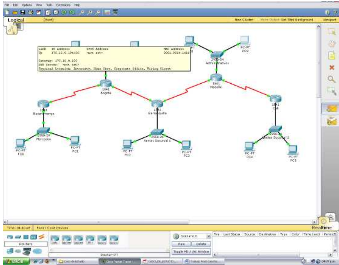
Fuente Simulador Packet Tracer
