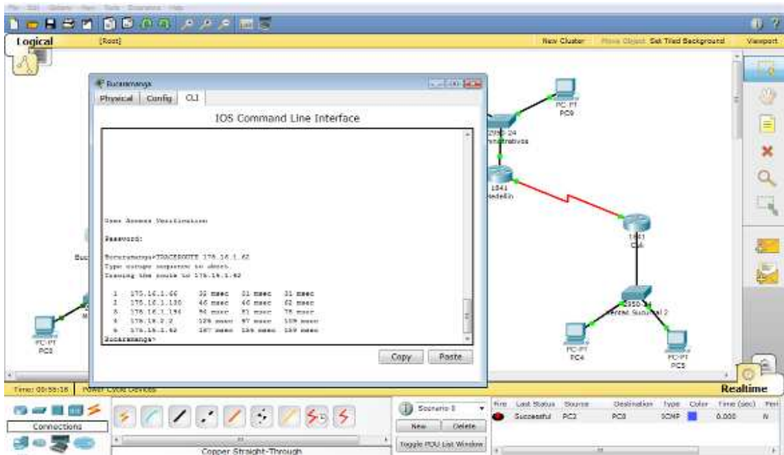
Figura 11 Prueba Uso Comando Traceroute.
