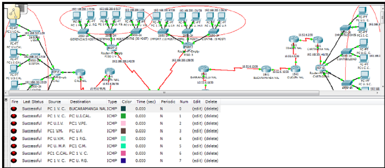
Figura 21 Estructura General.
