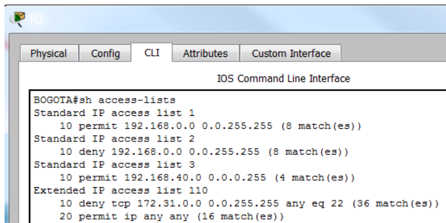
Figura 35. Listas de acceso configuradas en Router 2 para restringir acceso por SSH
