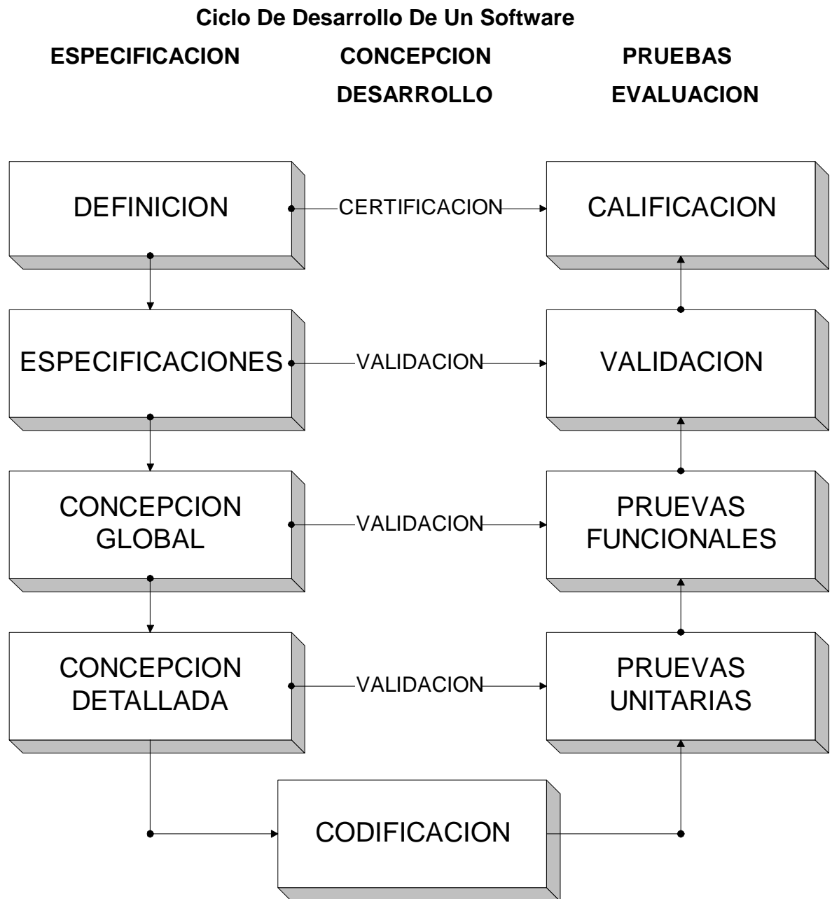
Fig. 9 Ciclo De Desarrollo De Un Software
