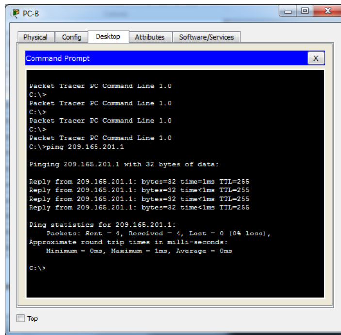
Ping del PC-B al R2
