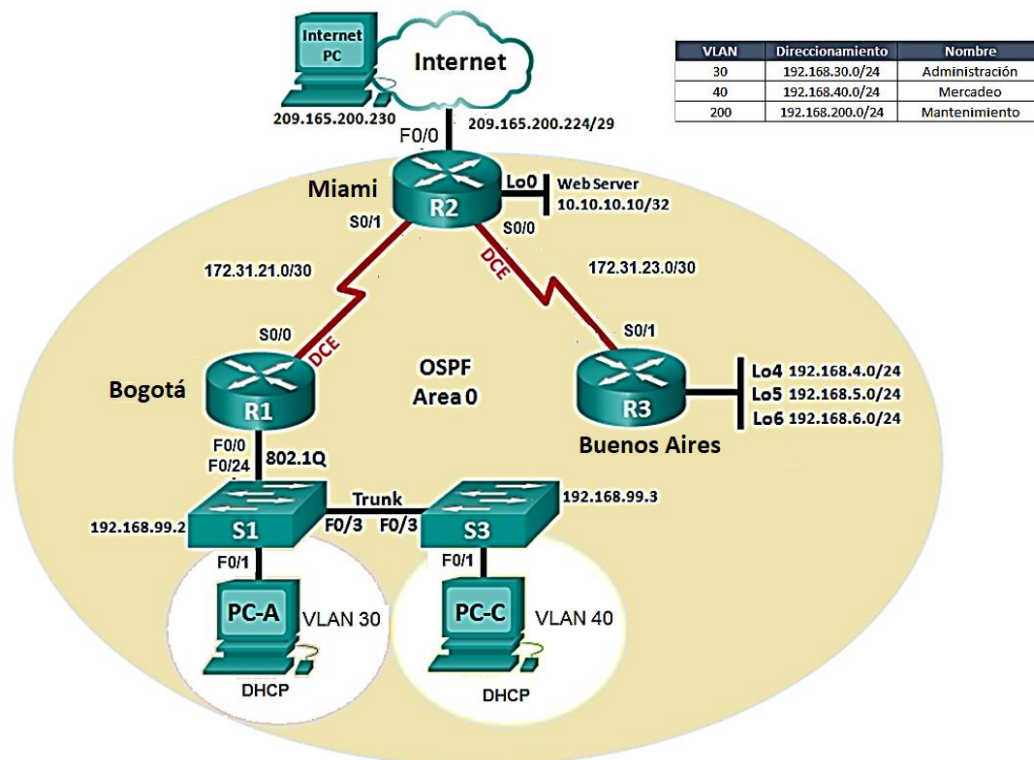
Ilustración 5 Topología
