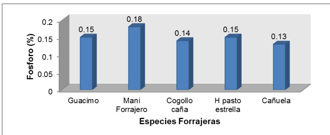
Figura N° 33. Promedio Fosforo.
