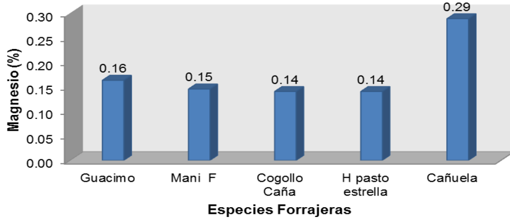
Figura N° 32. Promedio Magnesio.
