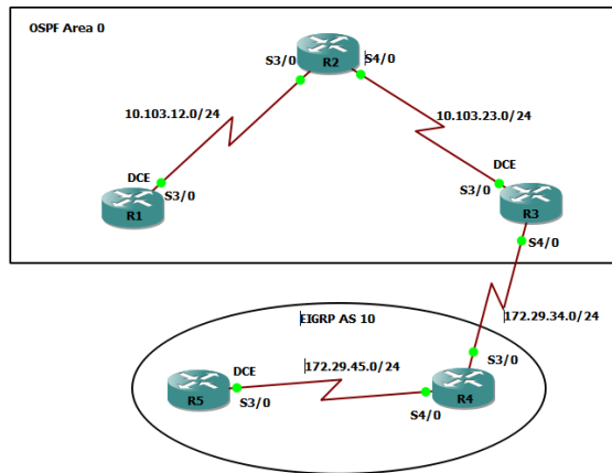
Figura 1. Topología de escenario 1.
