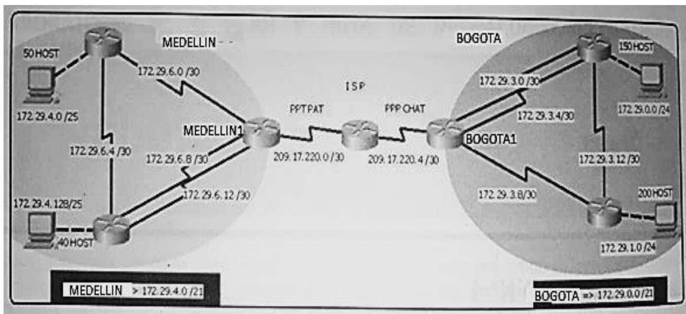
Ilustración 1 Topología escenario 1
