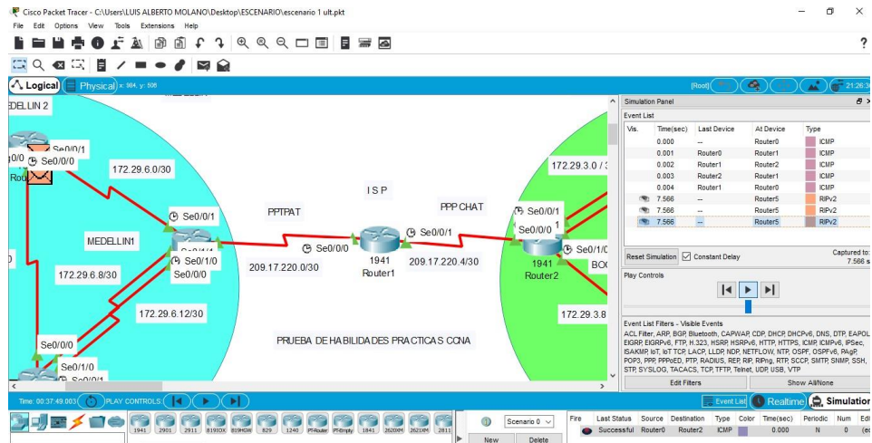
Ilustración 11 Router Bogotá 1 y Medellín 1 conectado por Route Rip,
