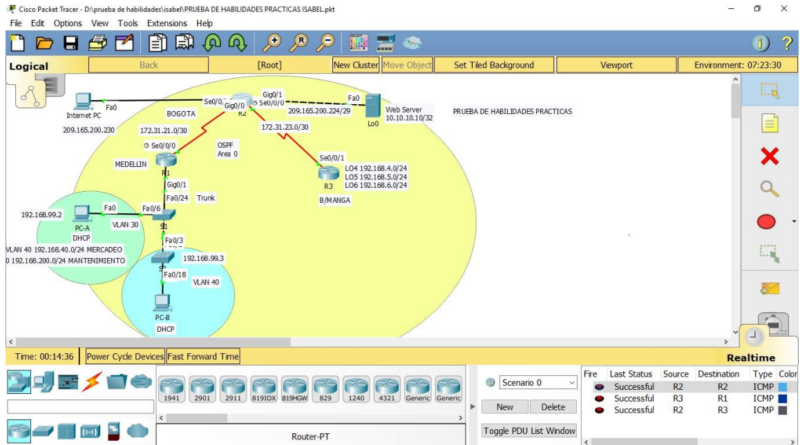
Ilustración 39 TOPOLOGIA
