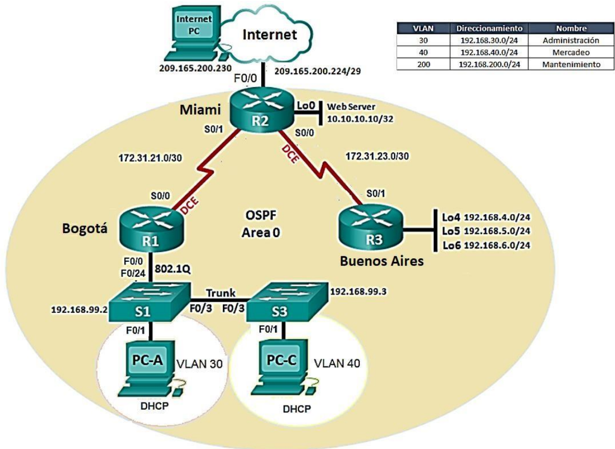
Ilustración 19 Escenario 2
