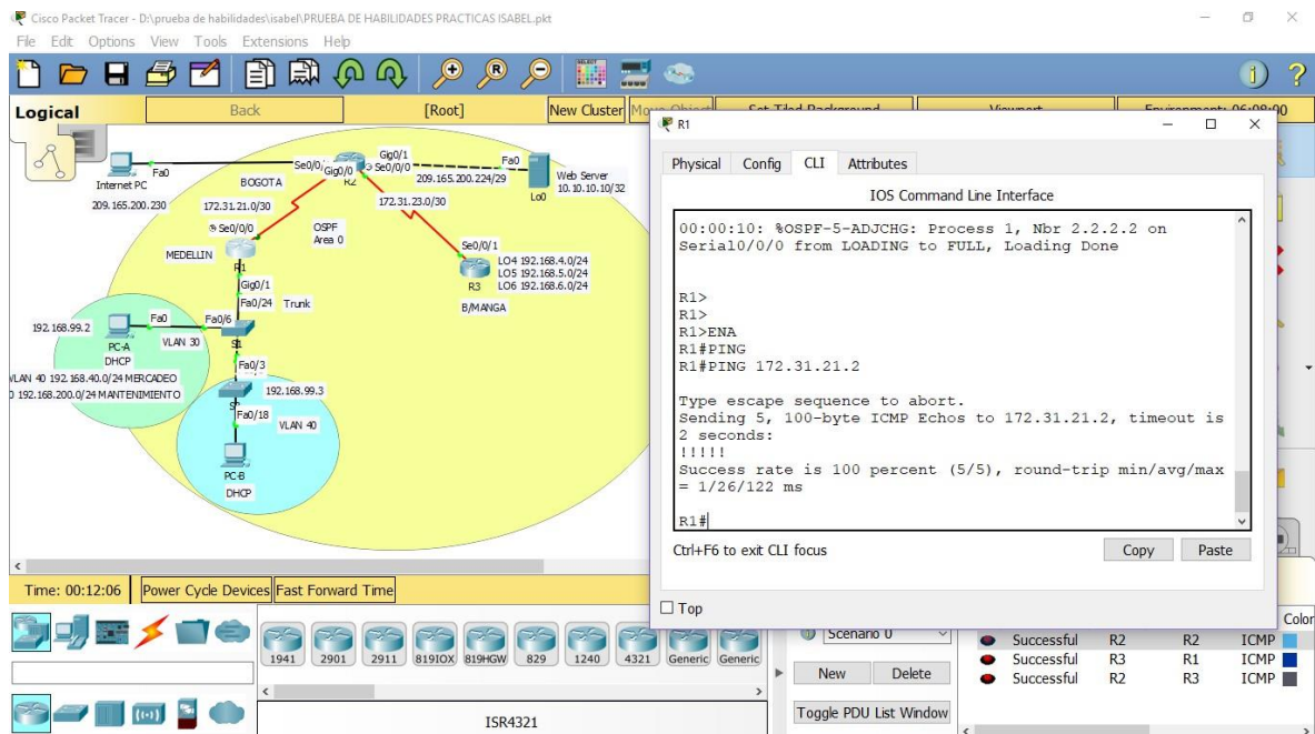
Ilustración 38 PING R2 A R3
