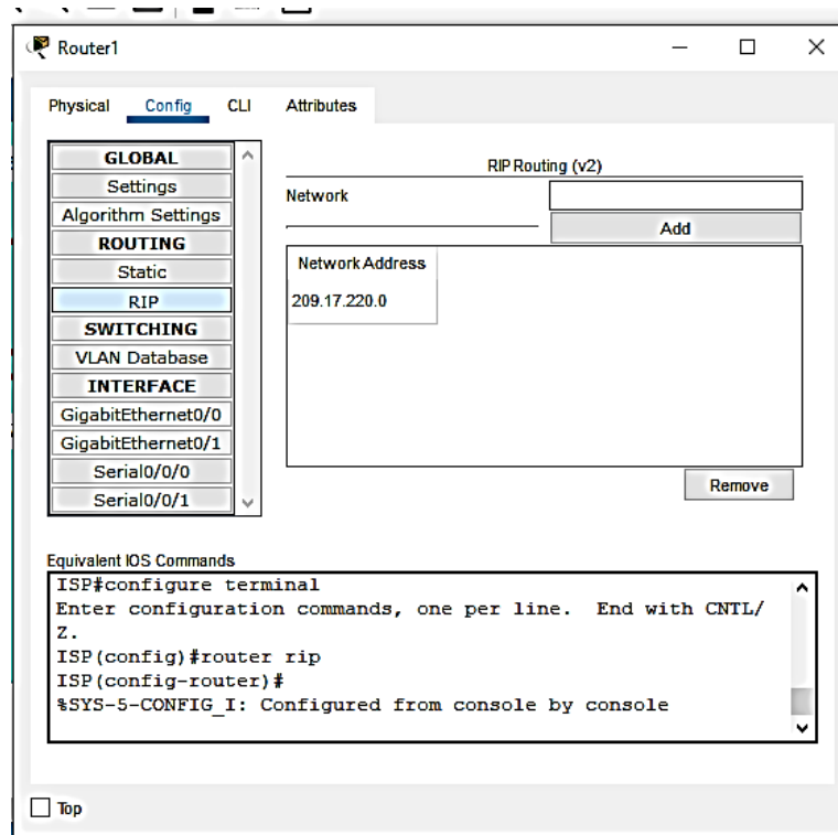
Ilustración 7 Configuration ISP de terminal 1.
