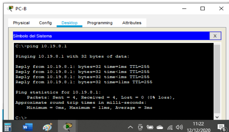
Figura 35. Ping desde PC-B a R1, G0/0/1.2 – Ipv4 10.19.8.1
