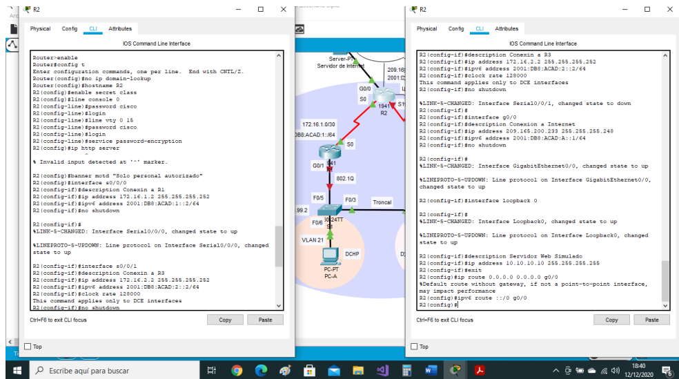
Figura 52. Configuración parámetros básicos en Router 2
