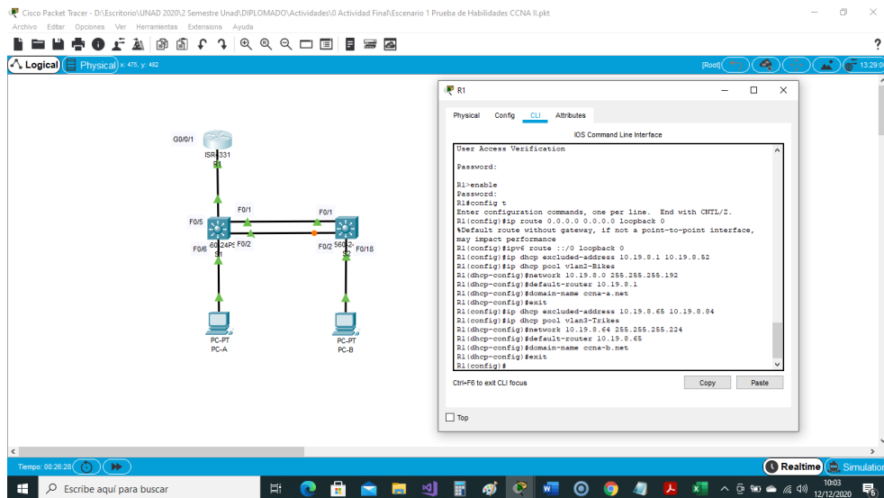
Figura 16. Configuración de soporte de host en Router
