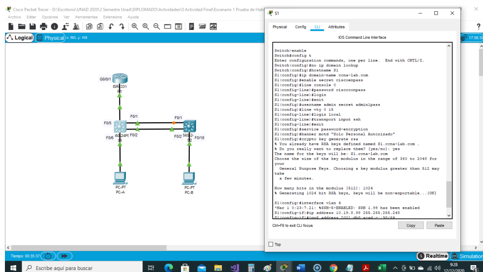
Figura 10. Configuración del Switch 1
