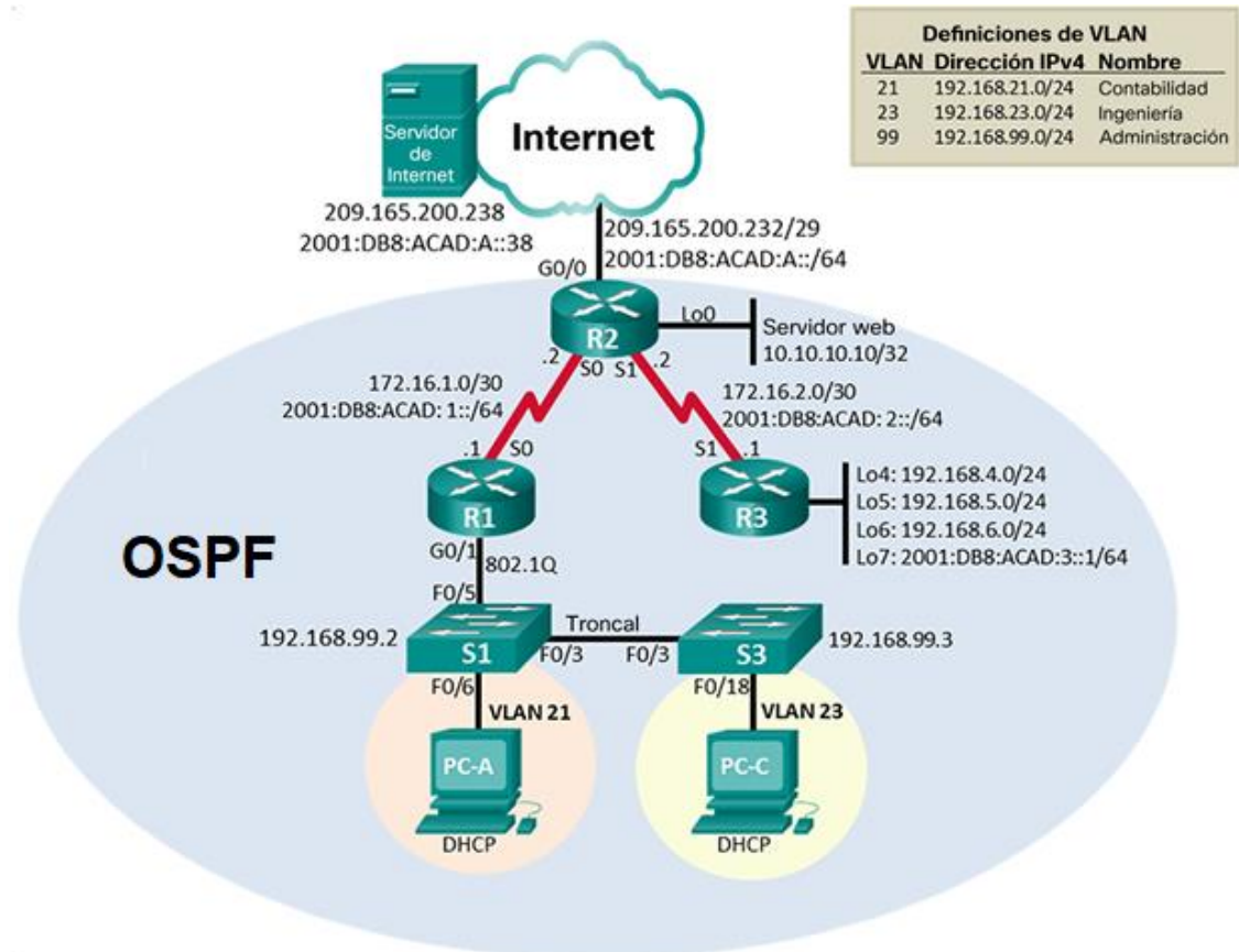
Figura 45. Topología escenario 2
