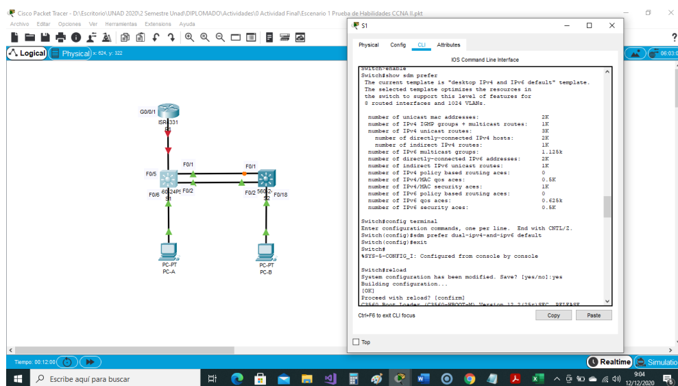
Figura 6. Configuración de plantilla SDM en Switch 1
