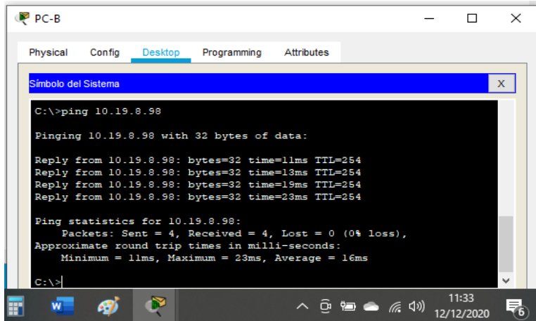
Figura 41. Ping desde PC-B a S1 VLAN4 – Ipv4 10.19.8.98
