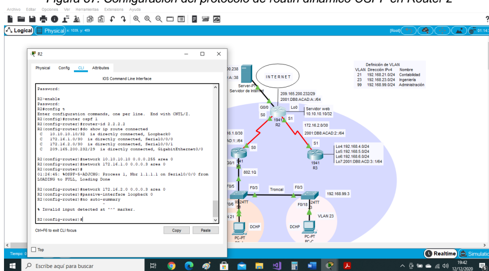
Figura 67. Configuración del protocolo de routing dinámico OSPF en Router 2
