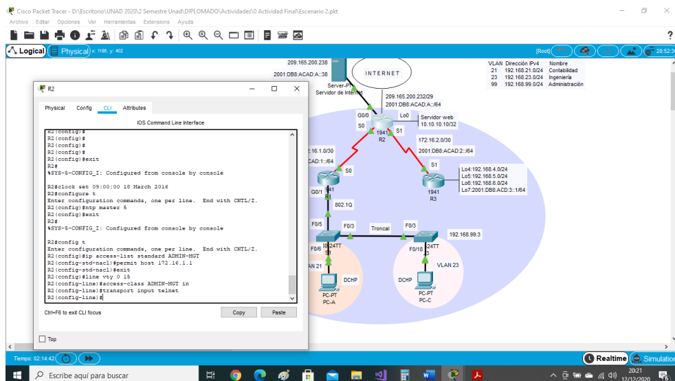
Figura 75. Restricción de acceso a líneas VTY en Router 2
