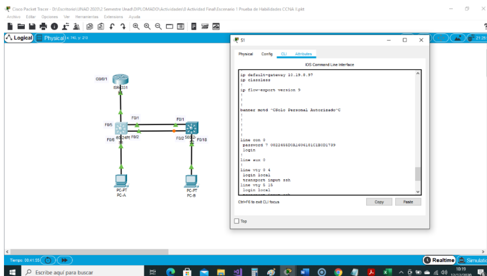
Figura 11. Verificación configuración Switch 1
