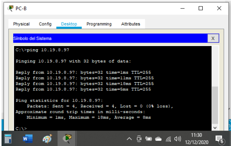
Figura 39. Ping desde PC-B a R1, G0/0/1.4 – Ipv4 10.19.8.97
