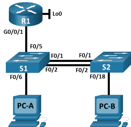
Figura 1. Topología escenario 1
