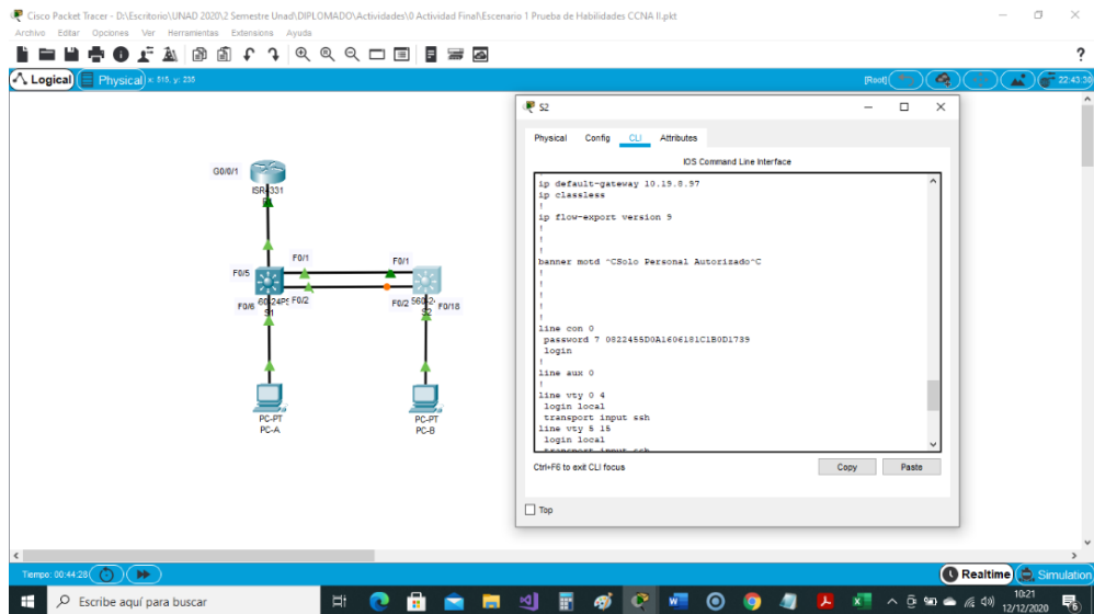
Figura 13. Verificación configuración Switch 2
