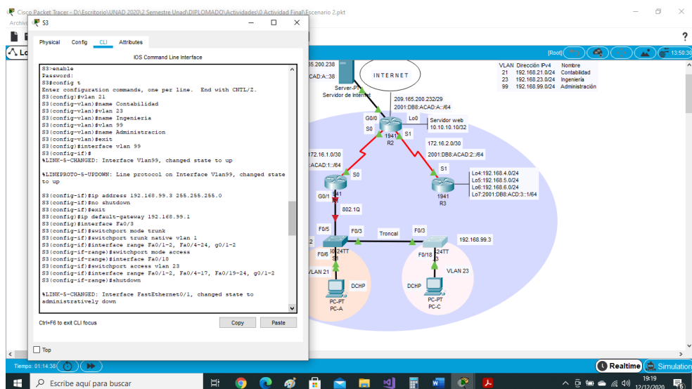
Figura 60. Configuración seguridad del switch 3, las VLAN y el routing entre VLAN.
