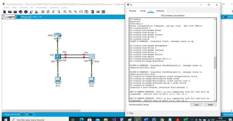
Figura 15. Configuración de la infraestructura de red (VLAN, Trunking, EtherChannel) en Switch 2
