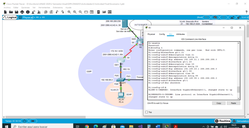
Figura 61. Configuración Subinterfaz 802.1Q en el Router 1
