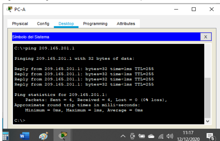
Figura 32. Ping desde PC-A a R1 Bucle 0 – Ipv6 2001:db8:acad:209::1
