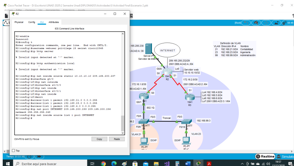
Figura 70. Configuración NAT estática y dinámica en Router 2
