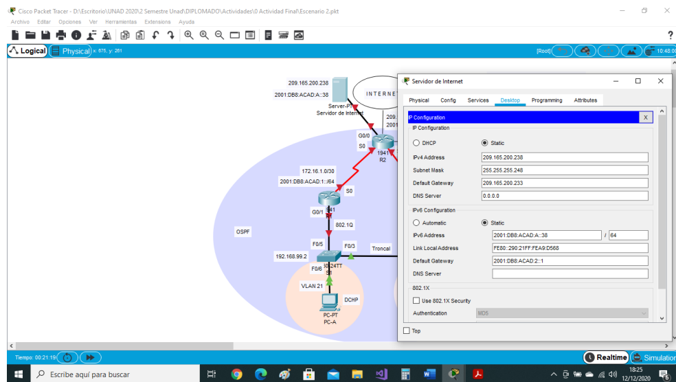
Figura 50. Configuración Servidor de Internet.
