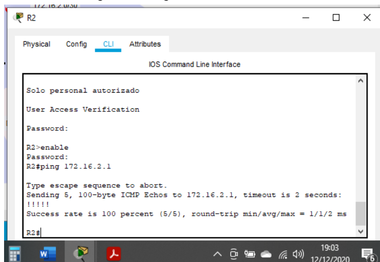
Figura 57. Ping desde R2 a R3 a la s0/0/1
