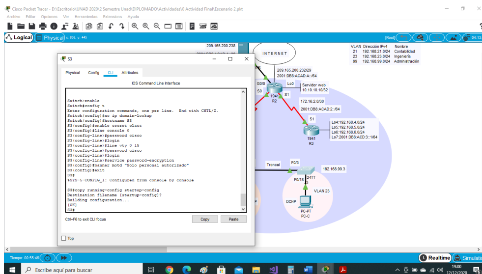
Figura 55. Configuración Switch 3
