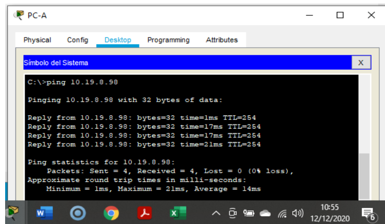
Figura 25. Ping desde PC-A a S1 VLAN4 – Ipv4 10.19.8.98
