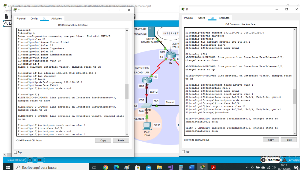
Figura 59. Configuración seguridad del switch 1, las VLAN y el routing entre VLAN.
