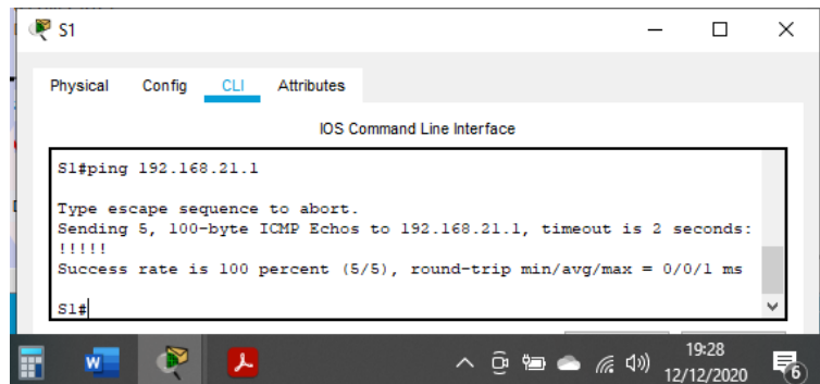
Figura 64. Desde Switch 1 ping a la dirección Vlan 21 de Router 1
