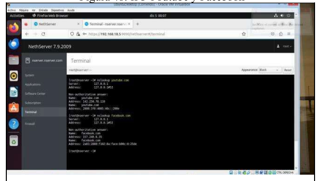
Figura 48. IPs Youtube y Facebook
