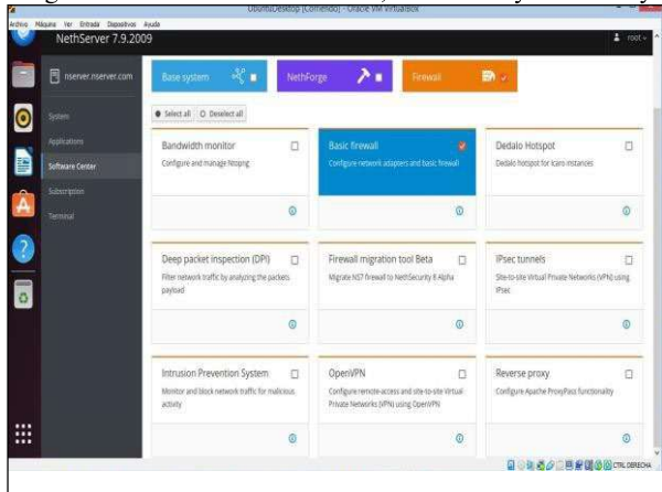
Figura 46. Instalación de Firewall, Web Filter y Web Proxy.
