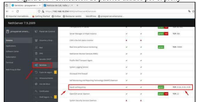
Figura 39. Verificación de puertos usados por el proxy
