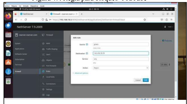
Figura 49. Regla para bloqueo YouTube
