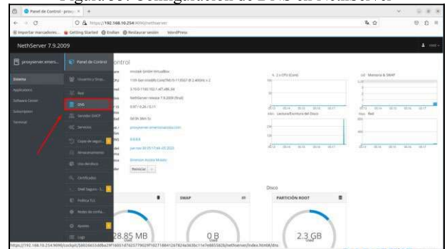
Figura 33. Configuración de DNS en NethServer
