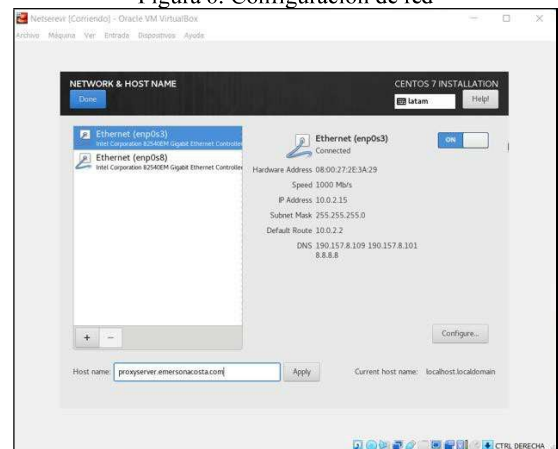
Figura 6. Configuración de red
