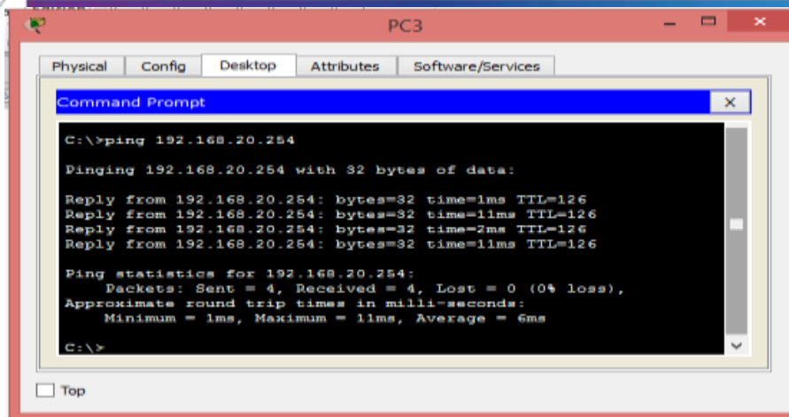
Figura 31. Conectividad exitosa en la PC3 hacia la red 192.168.20
