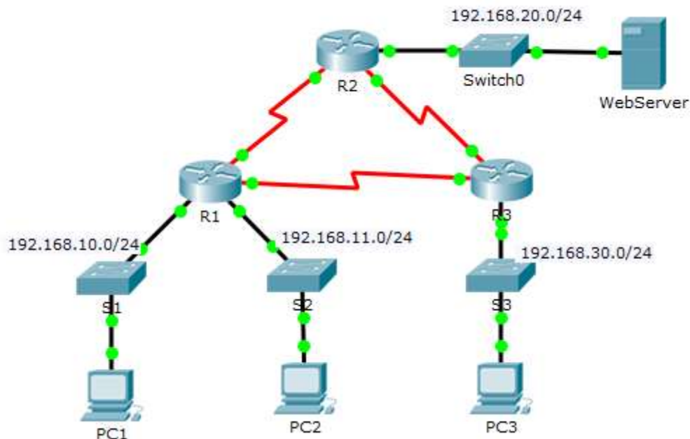
Figura 21. Topología
