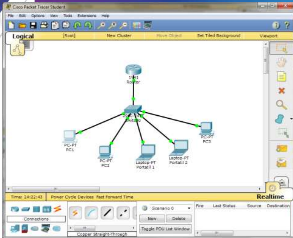
Configuración del router para que funcione con dhcp
