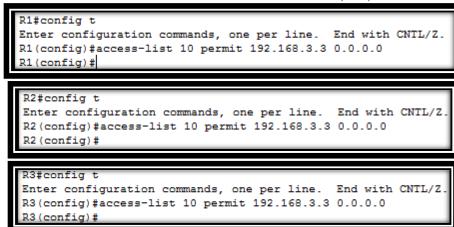
Figura 5. Configuración de las listas de acceso 10 para cada router
