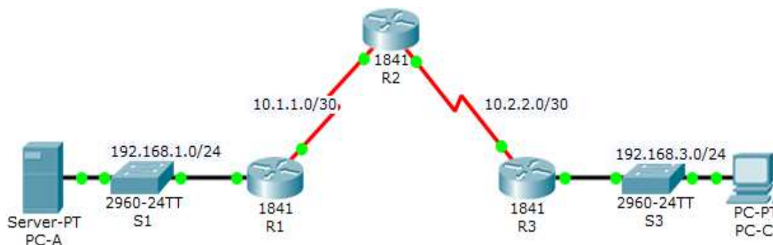
Figura 1. Topología
