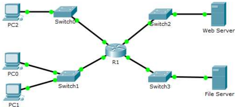
Figura 33. Topología
