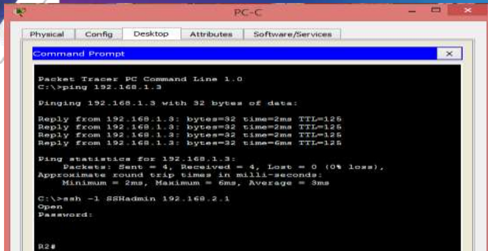
Figura 3. Verificación de ping y entrada SSH a R2 desde PC-C
