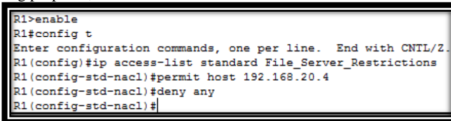
Figura 38. Configuración la ACL estándar con nombre en R1
