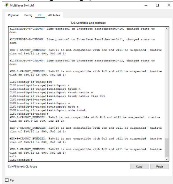
Ilustración 60. Configuración de los puertos como troncales en DLS2
