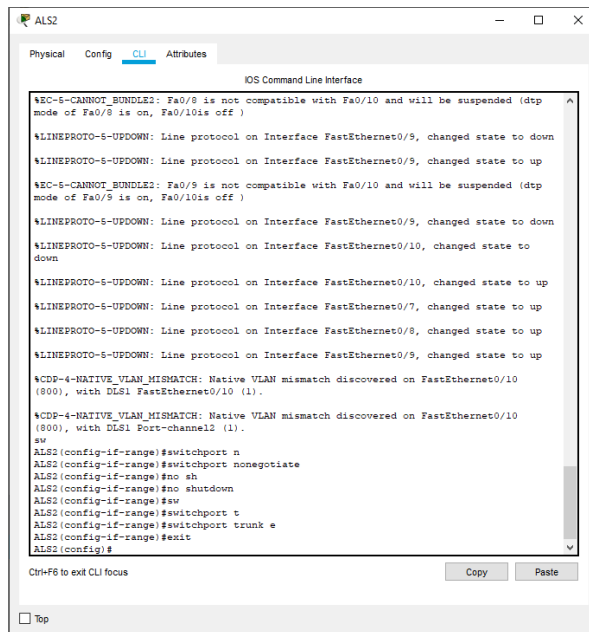
Ilustración 50. Configuración VLAN Nativa en ALS2
