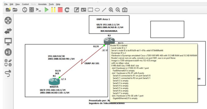
Ilustración 31. Consulta conectividad Router 2
