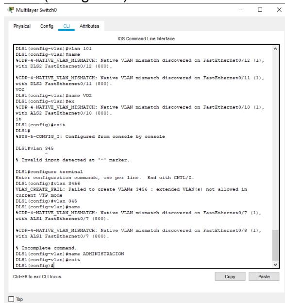
Ilustración 54. Configuración servidor principal de las VLAN NATIVA, EJECUTIVOS, HUESPEDES, VIDEONET en DLS1
