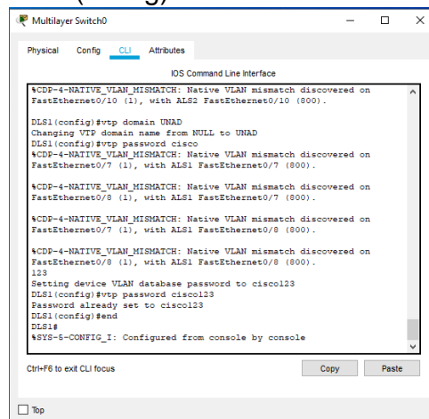
Ilustración 51. Configuración DLS1, ALS1 y ALS2 para utilizar VTP versión 3 en DLS1
