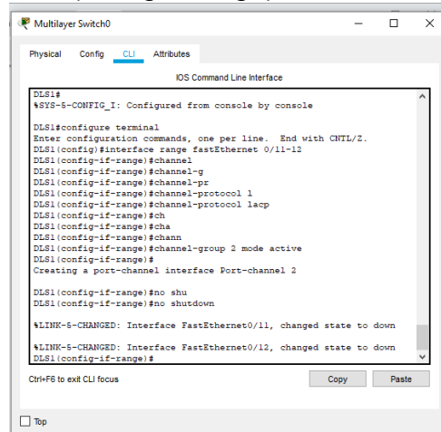
Ilustración 37. Configuración de puertos troncales y Port-channels en DLS1
