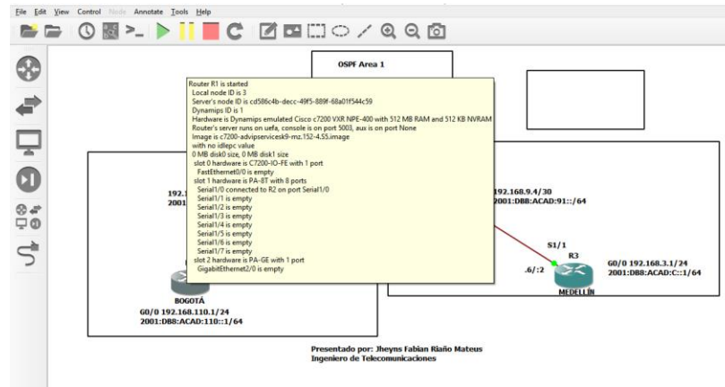
Ilustración 32. Consulta conectividad en Router 1
