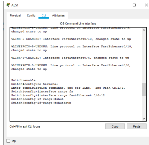
Ilustración 35. Apagado de Interfaces
