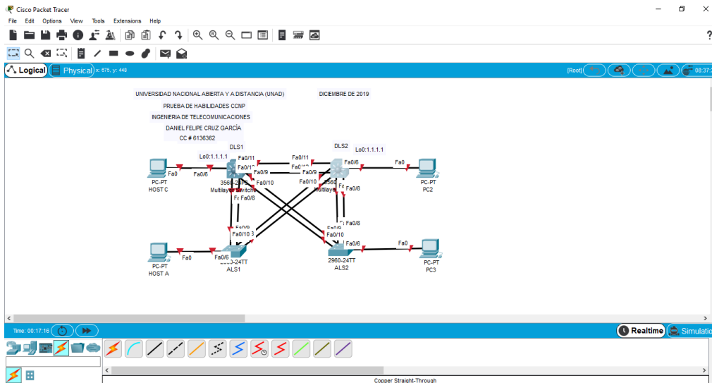
Ilustración 34. Topología Escenario 2 en simulador
