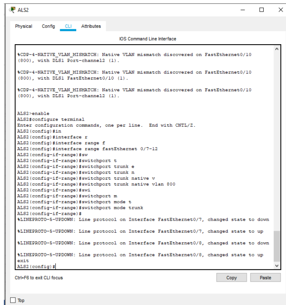
Ilustración 62. Configuración de los puertos como troncales en ALS2
