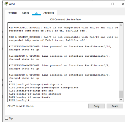
Ilustración 49. Configuración VLAN Nativa en ALS1
