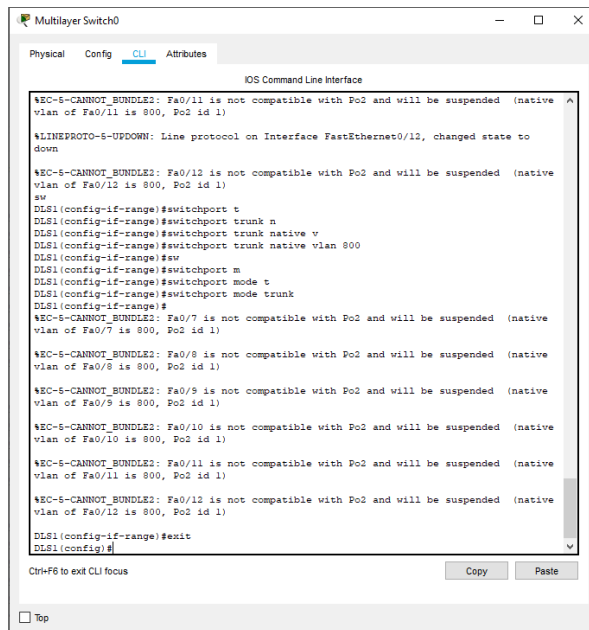
Ilustración 59. Configuración de los puertos como troncales en DLS1
