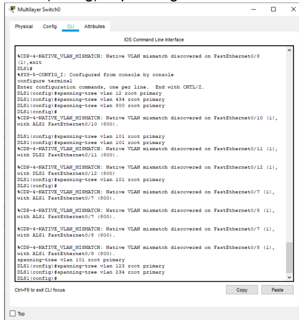
Ilustración 57. Configuración DLS1 como Spanning tree root para las VLAN en DLS1
