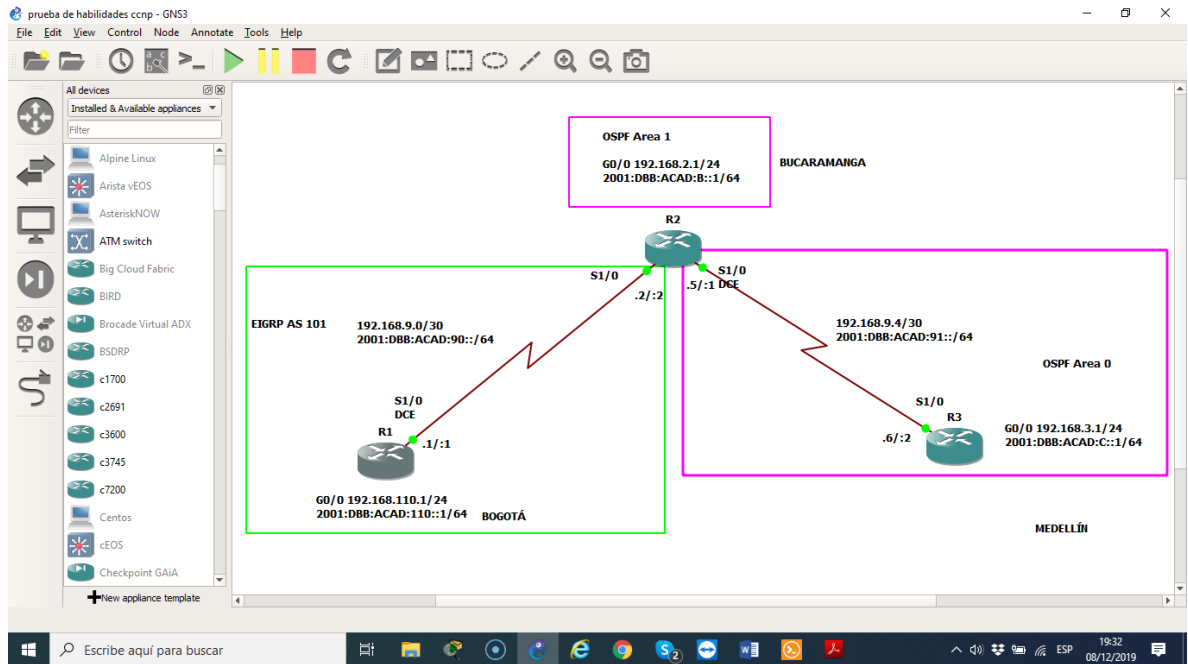
Ilustración 2. Topología de Red en Simulador
