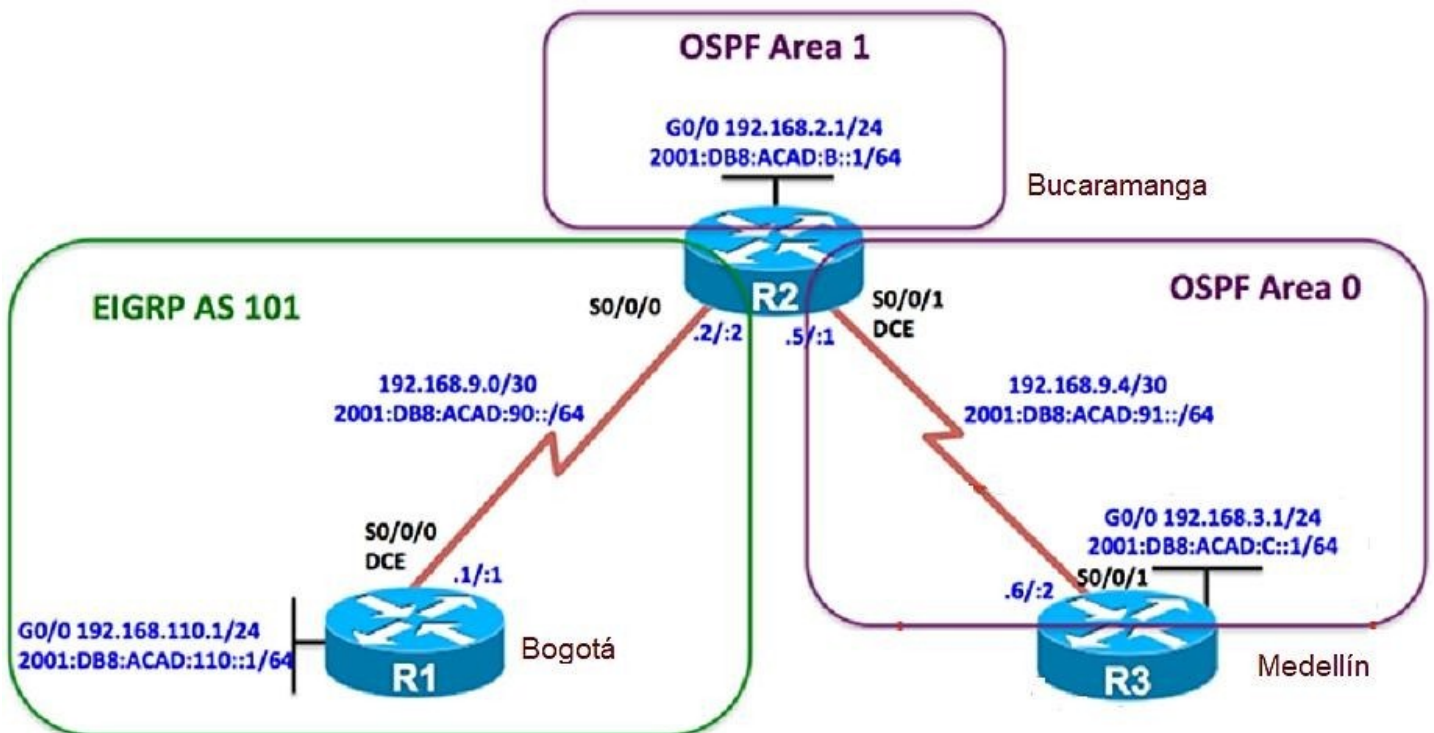
Imagen 1. Topología de red escenario 1
